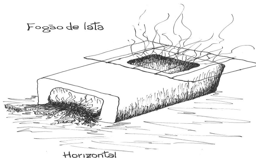
Figura 14 – Fogão de lata desenhado pelo professor Gilberto Kunz 20
