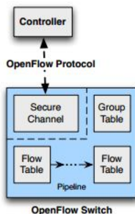
Figura 1.1 - Comunicação Controlador-Switch OpenFlow via canal seguro [12].
