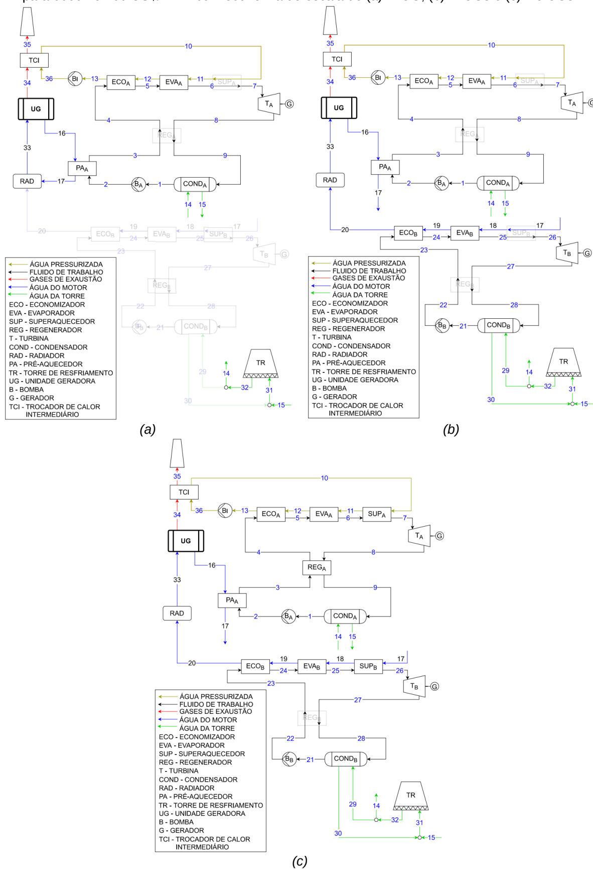
Figura 5.36 - Estrutura ótima ORC, utilizando água pressurizada, maximizando o lucro operacional para 6000h e 200 US$/MWh com economia de escala de (a). 1 UG, (b). 4 UGs e (c). 15 UGs.
