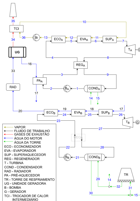
Figura 5.37 - Estrutura ótima ORC, utilizando vapor, maximizando o lucro operacional para 8000h e 150 US$/MWh com economia de escala de (a). 1 UG, (b). 4 UGs e (c). 15 UGs. (continuação)
