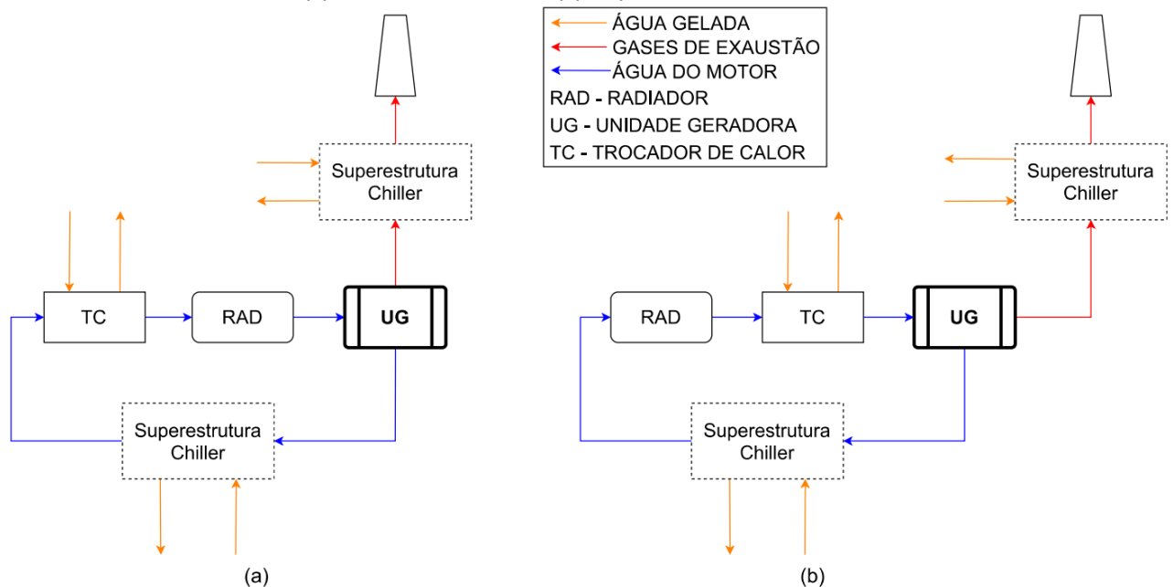
Figura 4.5 - Esquemático das possíveis posições do trocador de calor em conjunto com o radiador. (a) antes do radiador e (b) depois do radiador.
