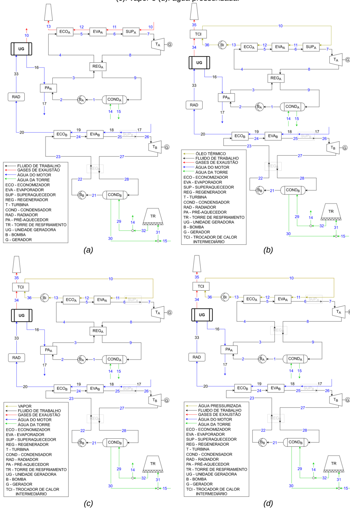
Figura 5.30 - Estrutura ótima ORC maximizando o lucro operacional para 8000h e 200 US$/MWh considerando como método de acoplamento (a). gases direto, (b). óleo térmico, (c). vapor e (d). água pressurizada.
