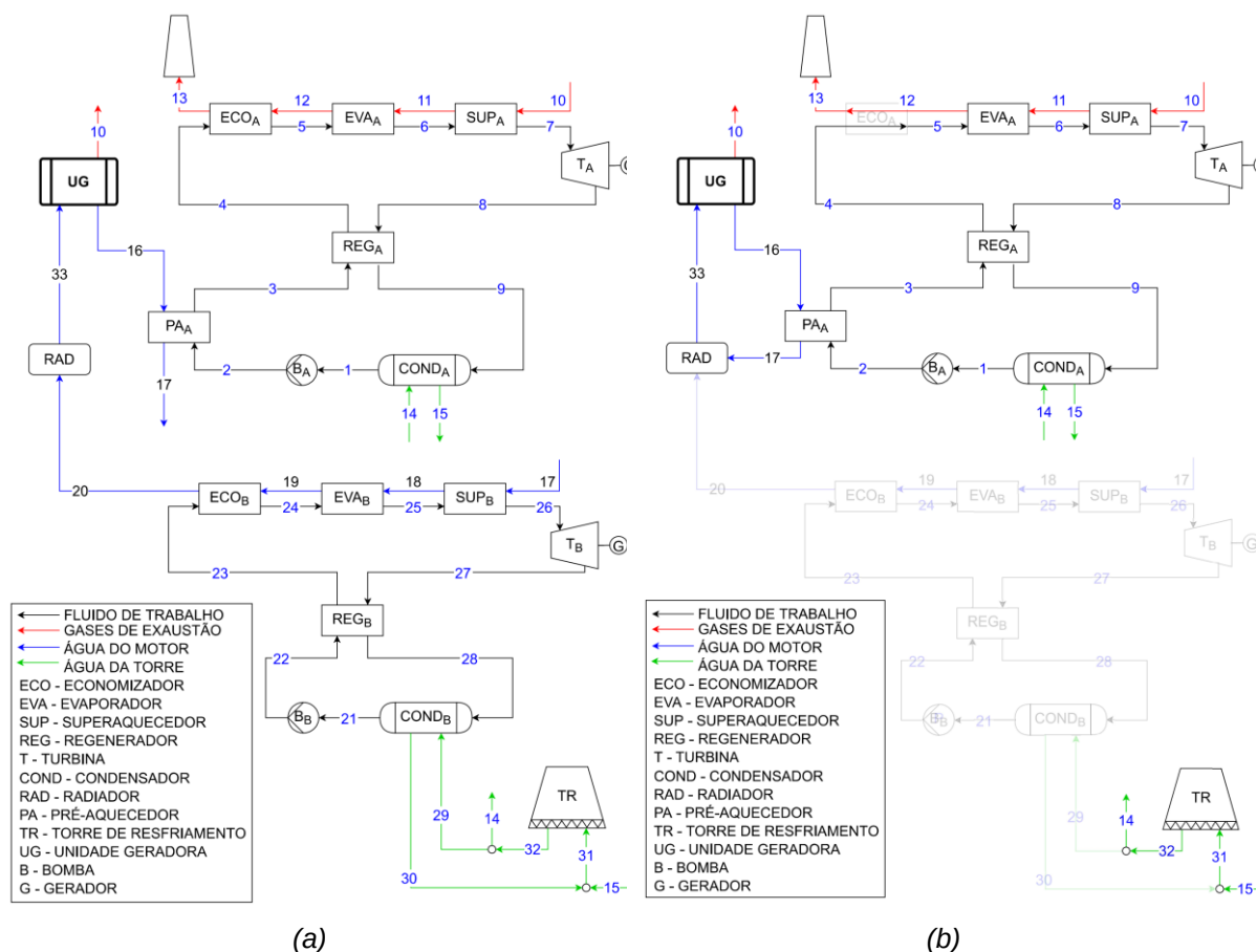
Figura 5.22 - Estrutura ótima ORC para motores sem caldeira considerando (a). maximização da potência líquida e (b). minimização do custo específico.
