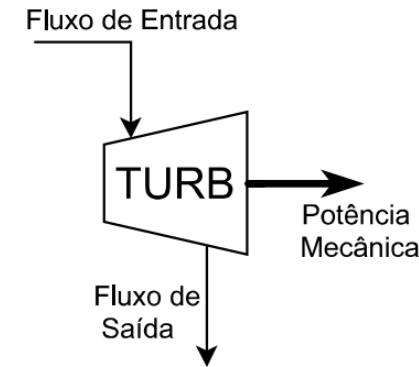
Figura 3.14 - Volume de controle de uma turbina genérica.
