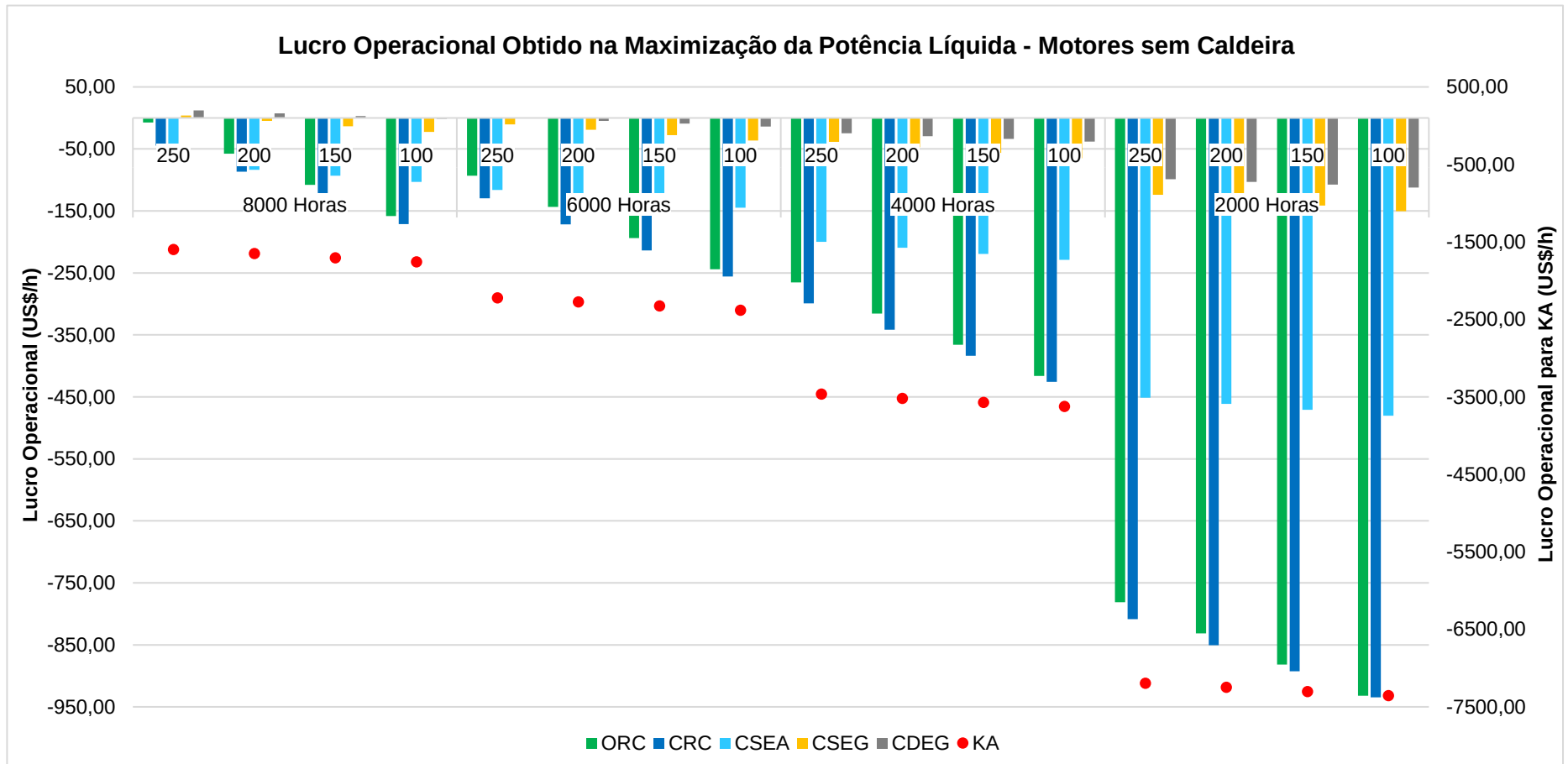
Figura 5.21 - Lucro operacional resultante da maximização da potência líquida para motores sem caldeira.
