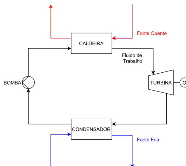
Figura 2.1 - Ciclo Rankine simples.
