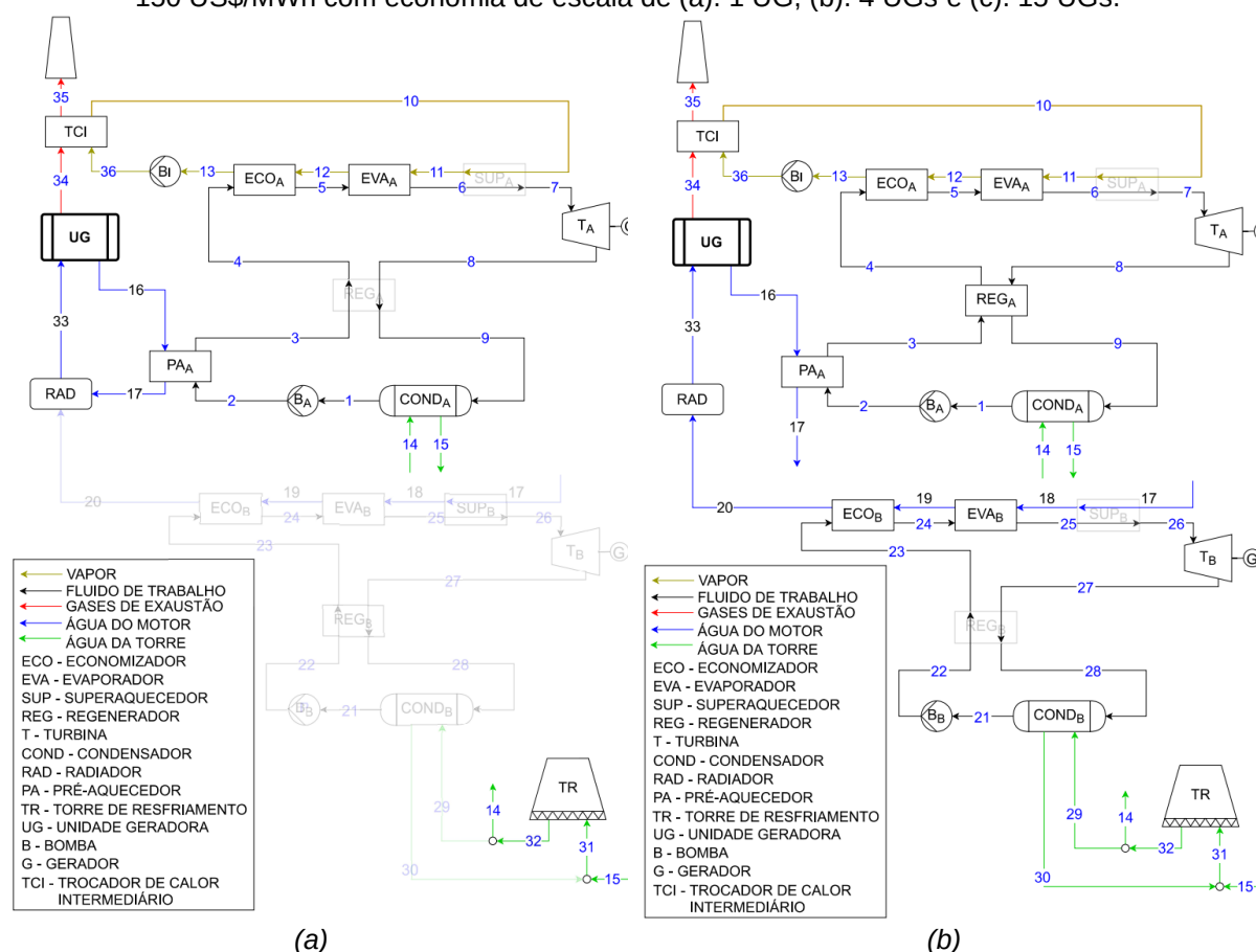
Figura 5.37 - Estrutura ótima ORC, utilizando vapor, maximizando o lucro operacional para 8000h e 150 US$/MWh com economia de escala de (a). 1 UG, (b). 4 UGs e (c). 15 UGs.
