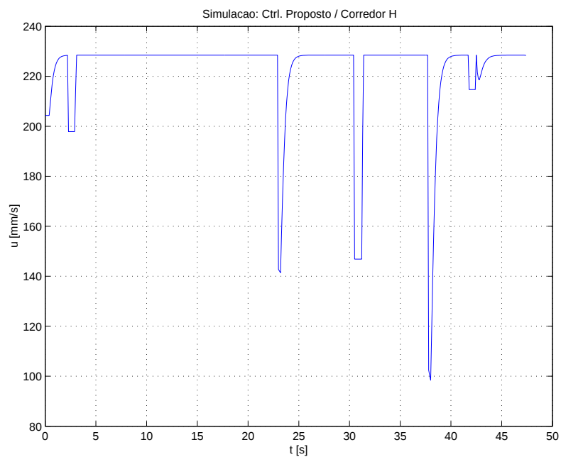
Figura 22: Velocidade linear do robô.
