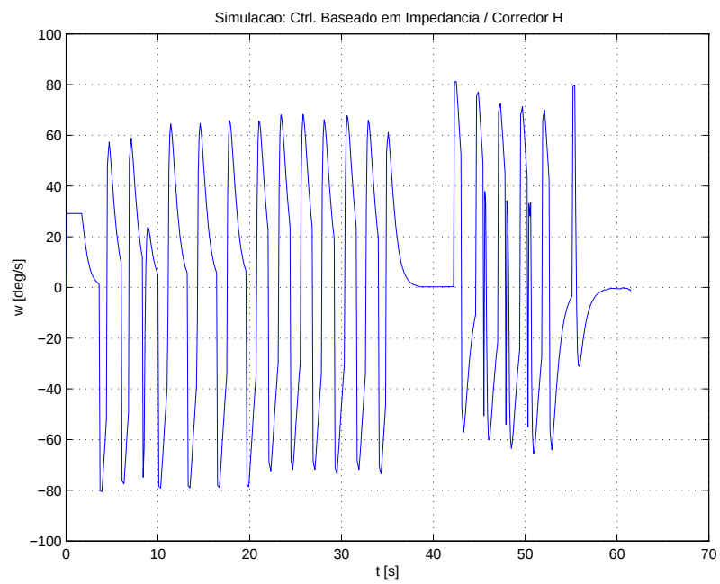
Figura 13: Velocidade angular do robô.
