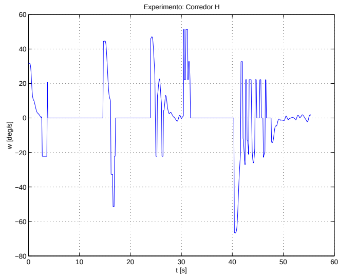
Figura 33: Velocidade angular \omega .
