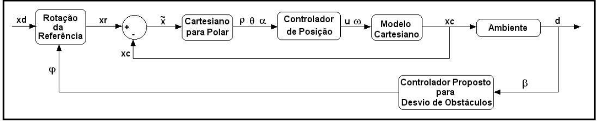
Figura 16: Diagrama de blocos para o sistema de controle proposto.
