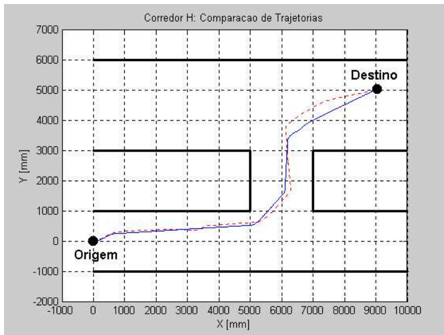
Figura 39: Posição do robô. Linha tracejada: experimento. Linha contínua: simulação
