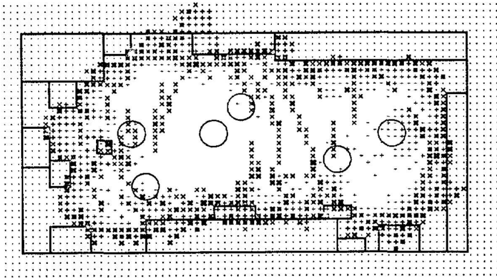
Figura 1: Mapa 2D gerado com o método Certainty Grid [5].
