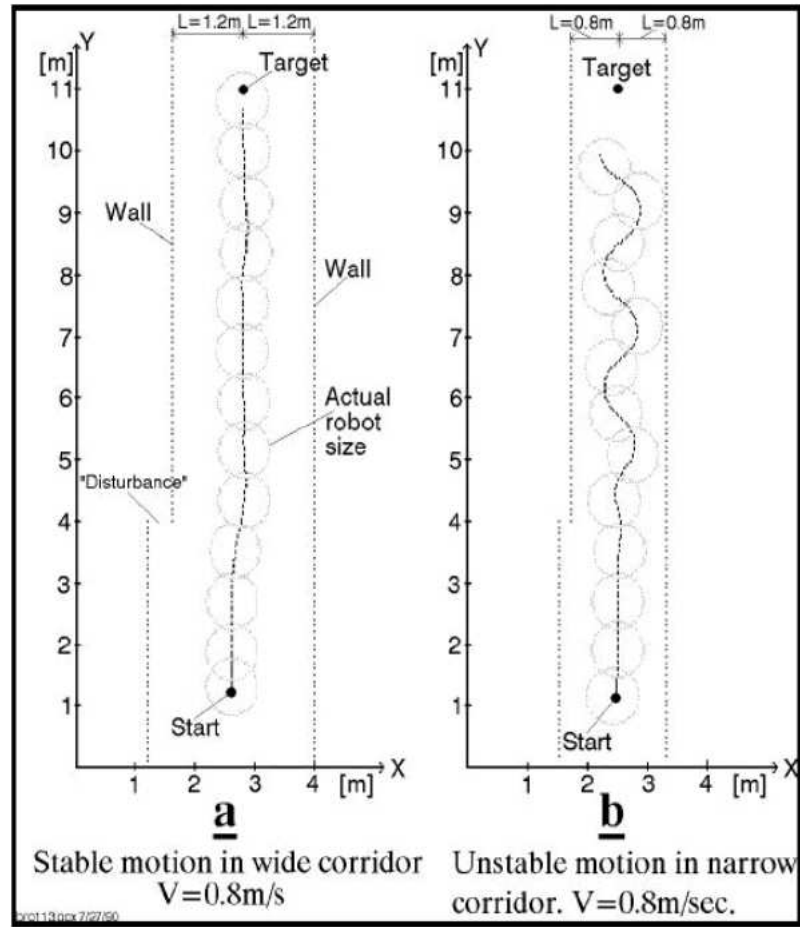
Figura 3: Problema do VFF com corredores estreitos [15].
