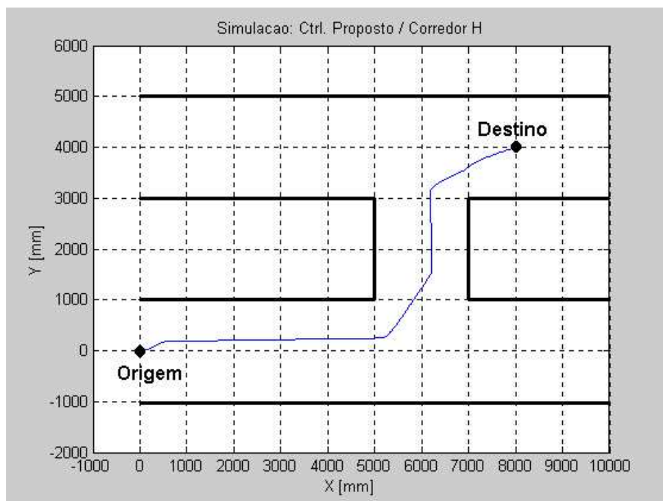
Figura 21: Trajetória do robô.
