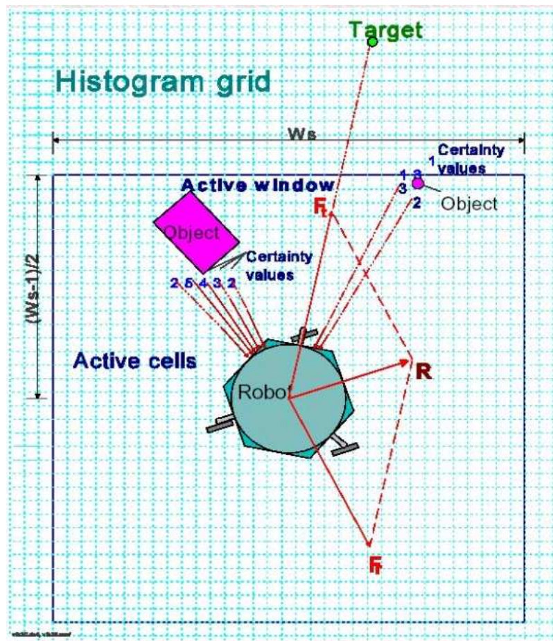
Figura 2: Método do Campo de Forças Virtuais [16].
