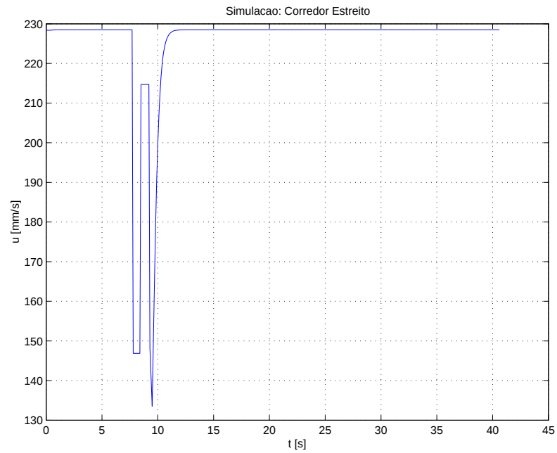
Figura 18: Velocidade linear do robô no corredor estreito.
