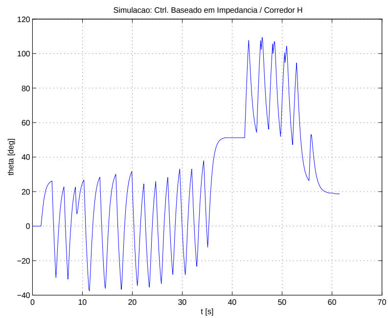
Figura 14: Orientação do robô.
