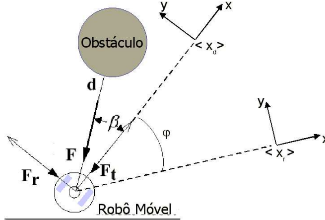
Figura 10: Detecção do obstáculo e a força fictícia gerada.
