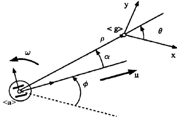
Figura 6: Diagrama para obtenção do modelo cinemático do robô.
