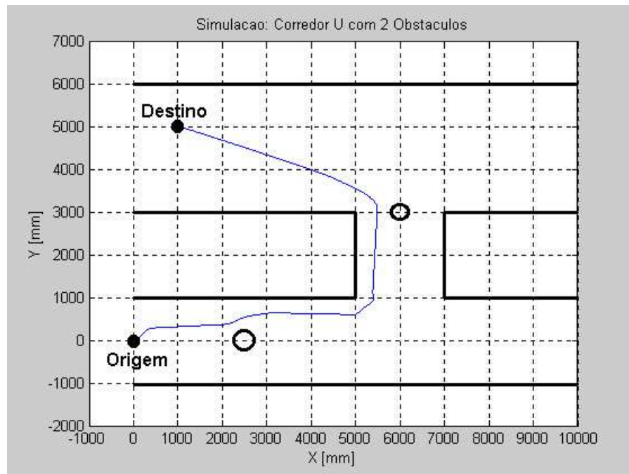
Figura 41: Simulação utilizando o controlador proposto.
