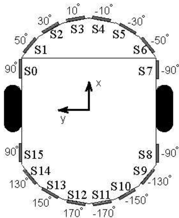
Figura 28: Distribuição dos sonares no robô PIONEER 2-DX .
