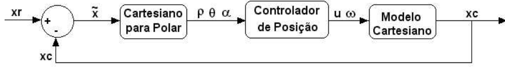
Figura 8: Diagrama de blocos do controlador de posição final.
