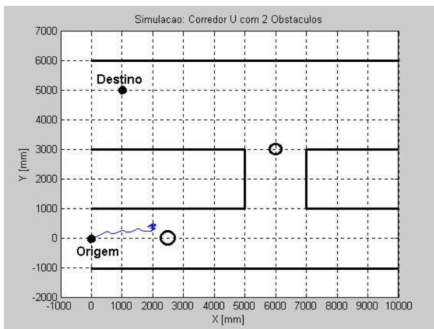
Figura 42: Simulação utilizando o controlador baseado em impedância.
