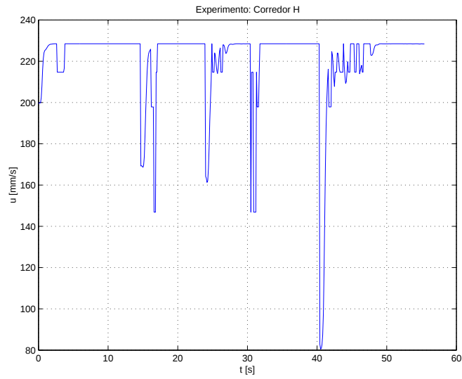
Figura 32: Velocidade linear u .
