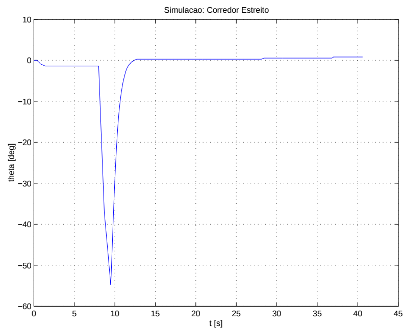
Figura 20: Orientação do robô no corredor estreito.
