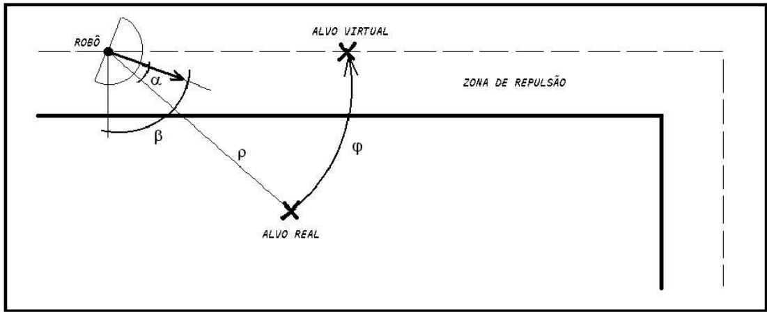
Figura 15: Obtenção do ângulo \varphi .
