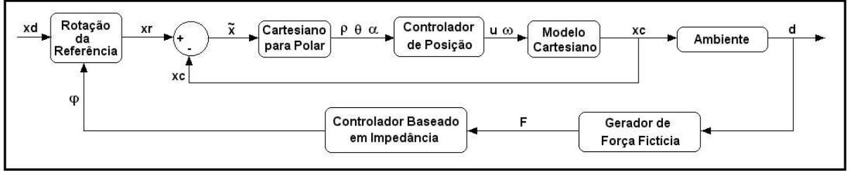
Figura 9: Diagrama de blocos para o sistema de controle baseado em impedância.
