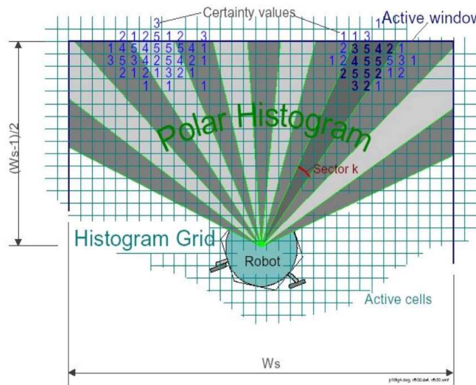
Figura 4: Mapeamento dos setores para o histograma polar [17].
