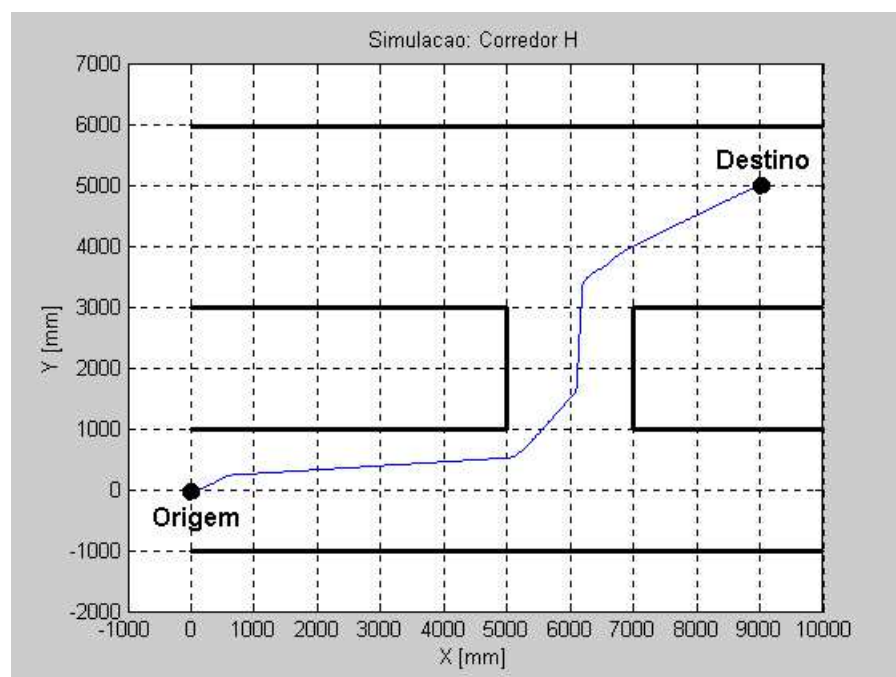
Figura 35: Trajetória do robô.
