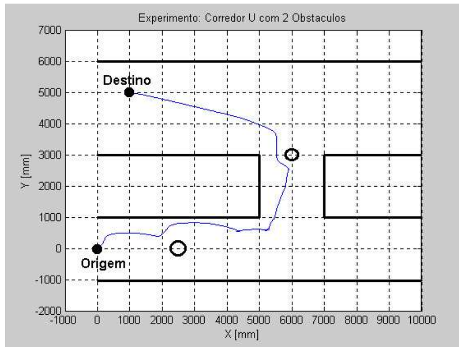
Figura 40: Experimento utilizando o controlador proposto.
