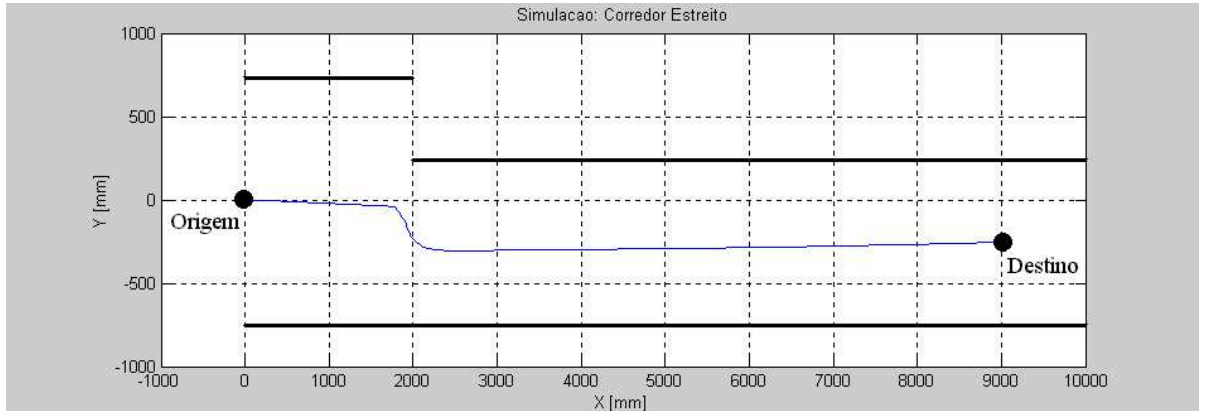
Figura 17: Trajetória do robô ao longo do corredor estreito.
