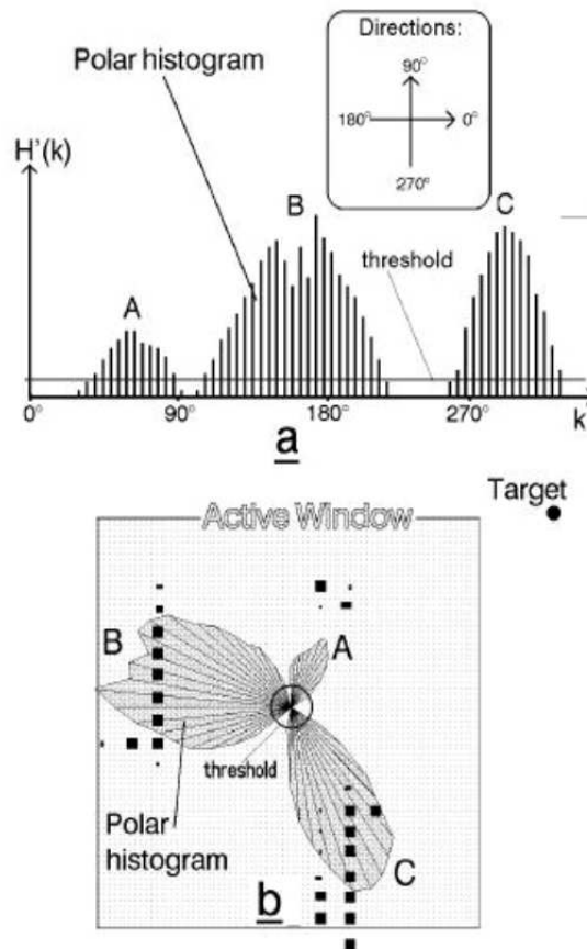
Figura 5: Histogramas polares de densidade de obstáculos [17].
