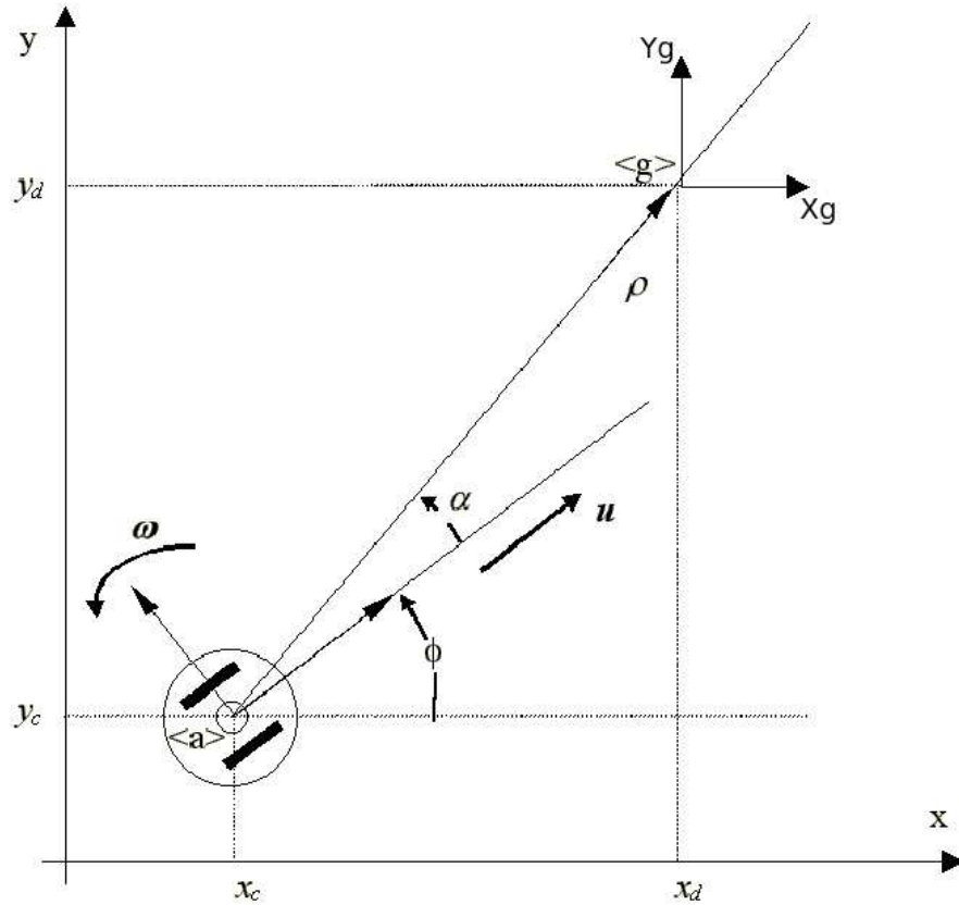
Figura 7: Erros de posição e orientação do robô em relação ao alvo.
