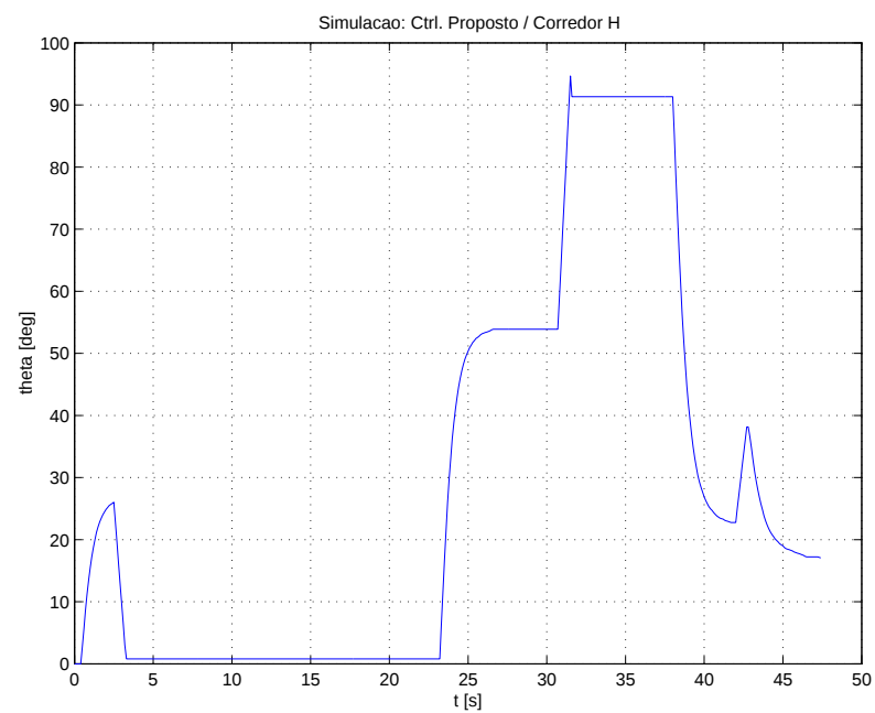
Figura 24: Orientação do robô.
