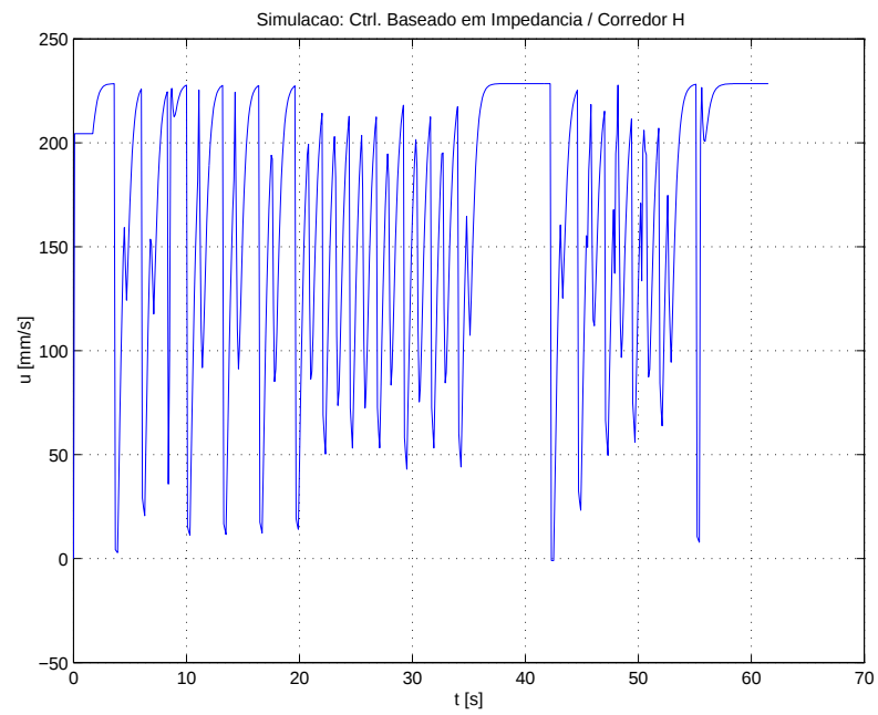
Figura 12: Velocidade linear do robô.
