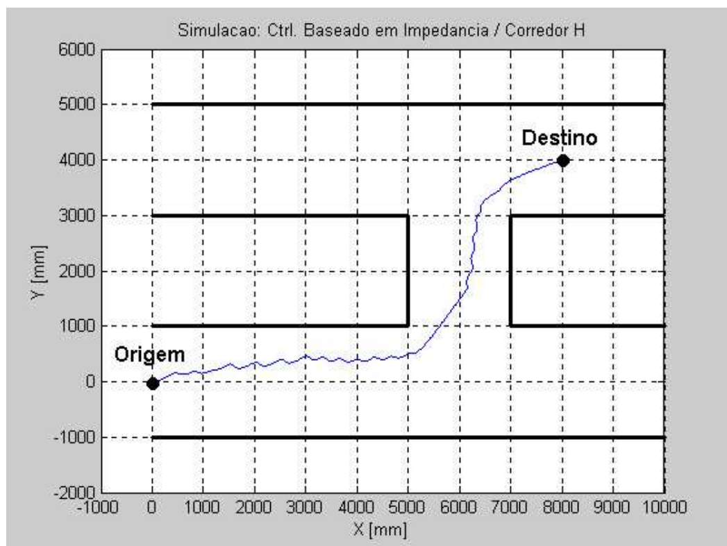
Figura 11: Trajetória do robô.
