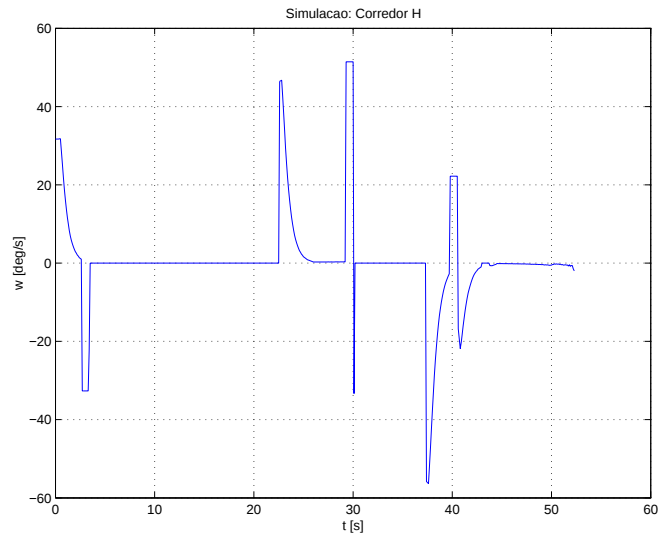
Figura 37: Velocidade angular \omega .
