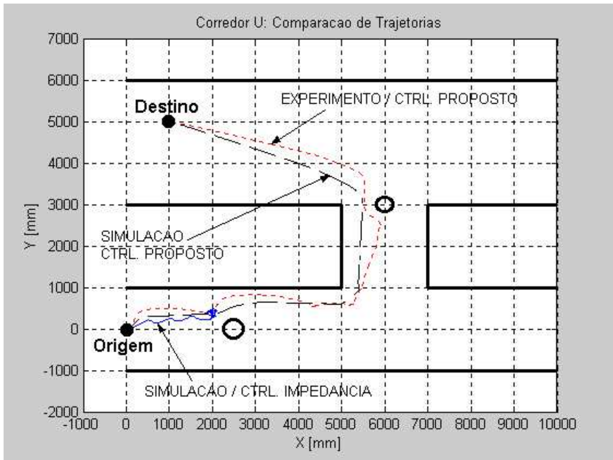
Figura 43: Comparação dos resultados.
