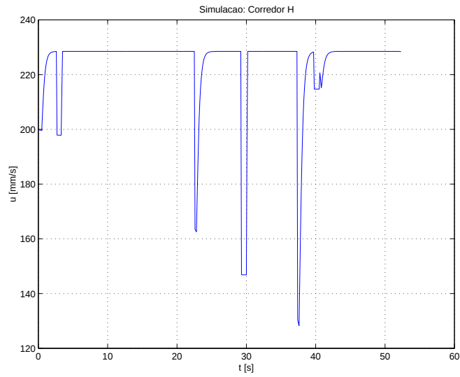
Figura 36: Velocidade linear u .
