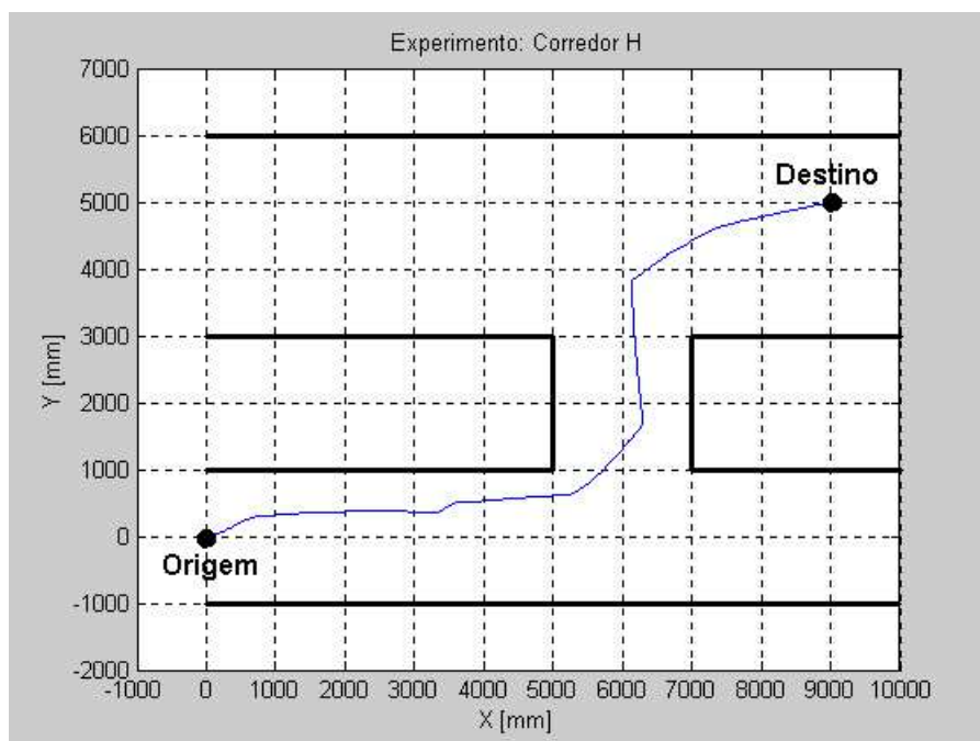
Figura 31: Trajetória do robô.
