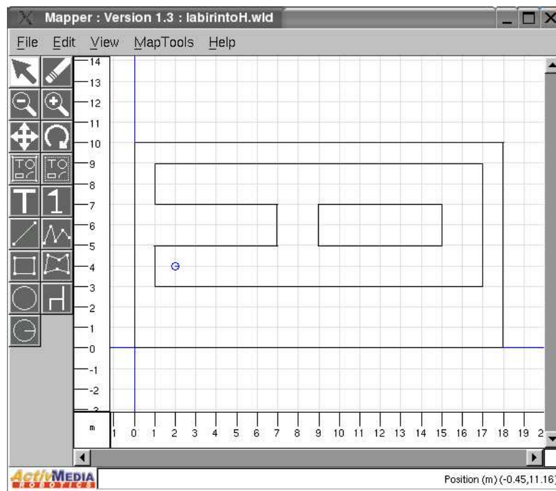
Figura 26: Mapper : Ferramenta para criação/edição de mapas.
