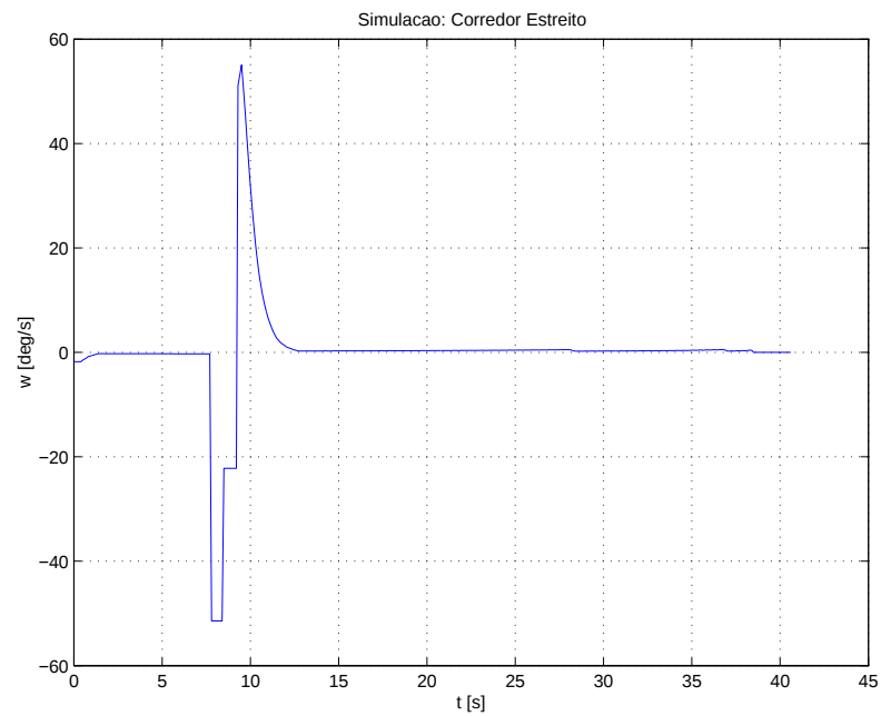
Figura 19: Velocidade angular do robô no corredor estreito.
