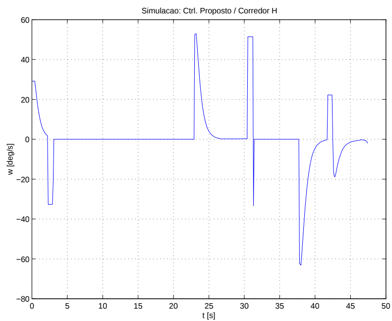
Figura 23: Velocidade angular do robô.
