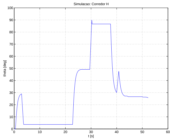
Figura 38: Orientação do robô.
