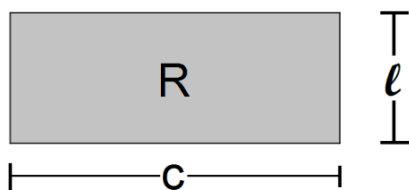
Figura 23: Retângulo R de comprimento c e largura \ell
