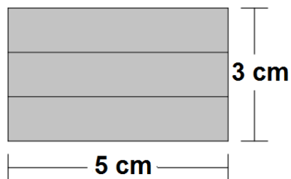
Figura 20: Retângulo de lados 5 cm e 3 cm dividido em 5 retângulos iguais
