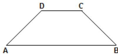
Figura 12: Trapézio ABCD
