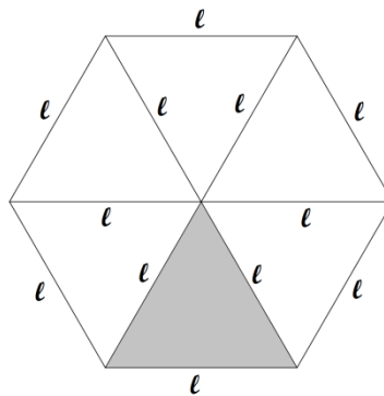
Figura 36: Hexágono regular de lado \ell dividido em 6 triângulos equiláteros
