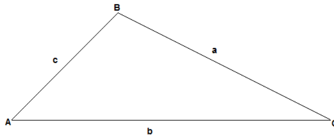
Figura 32: Triângulo de lados a , b e c
