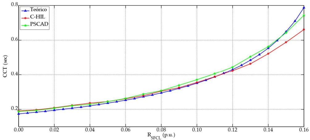
Gráfico 16 - Comparação entre tempos críticos de falta: CCT teórico (azul), PSCAD (verde) e C-HIL (vermelho).
