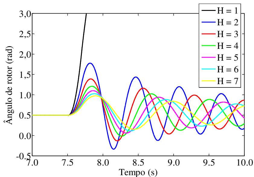
Gráfico 7 - Curvas de oscilação do VSG para diferentes valores de H .
