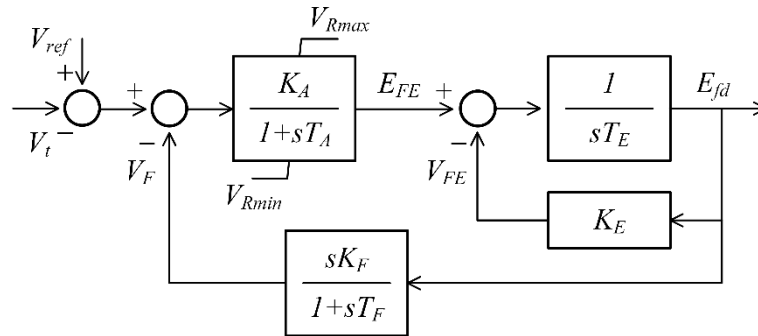
Figura 8 - Diagrama do sistema de excitação DC1A modificado utilizado
