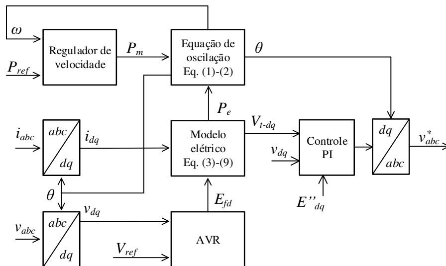
Figura 2 - Diagrama de controle em referencial dq de uma máquina síncrona virtual.
