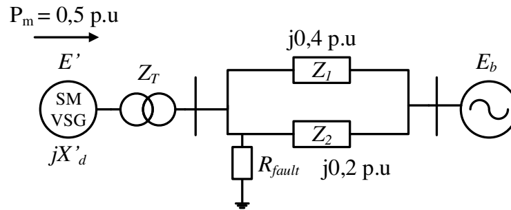
Figura 14 - Situação do sistema no instante anterior a uma alteração de topologia.
