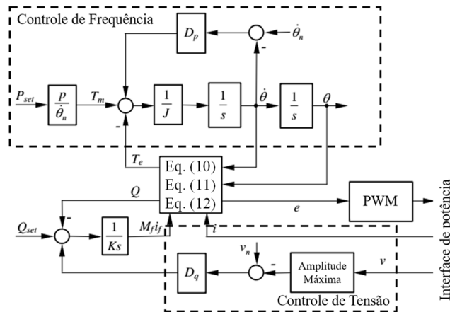
Figura 3 - Diagrama de controle utilizado na implementação da topologia Synchronverter .
