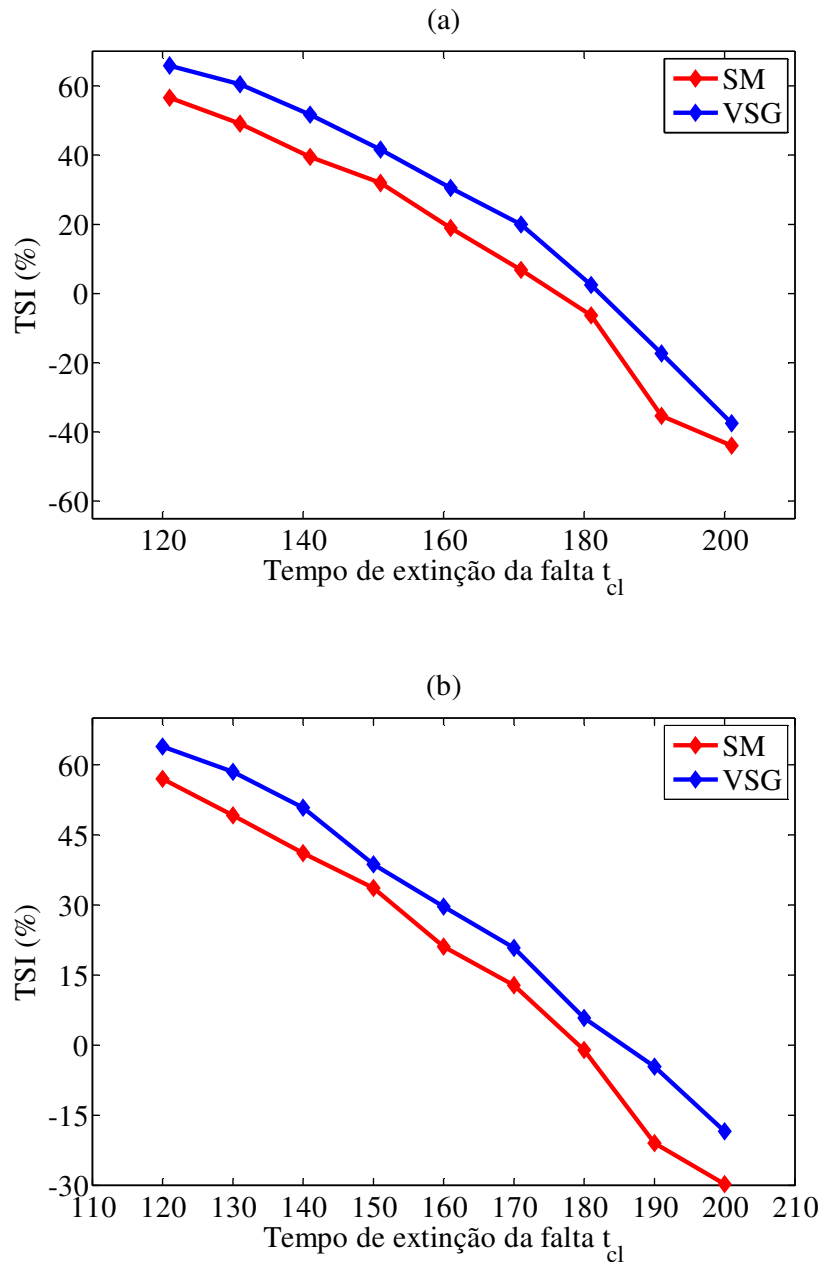
Gráfico 4 - Variação do TSI em função do tempo de extinção de falta para os Cenários 1 (a) e 5 (b).
