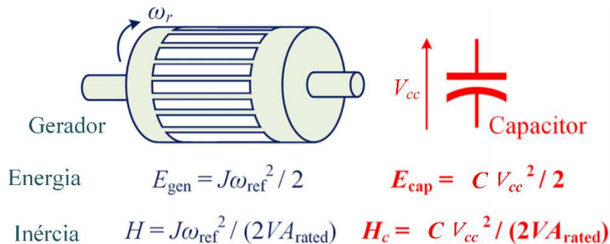
Figura 12 - Analogia entre a energia armazenada no elo CC do inversor e a energia rotacional de uma MS
