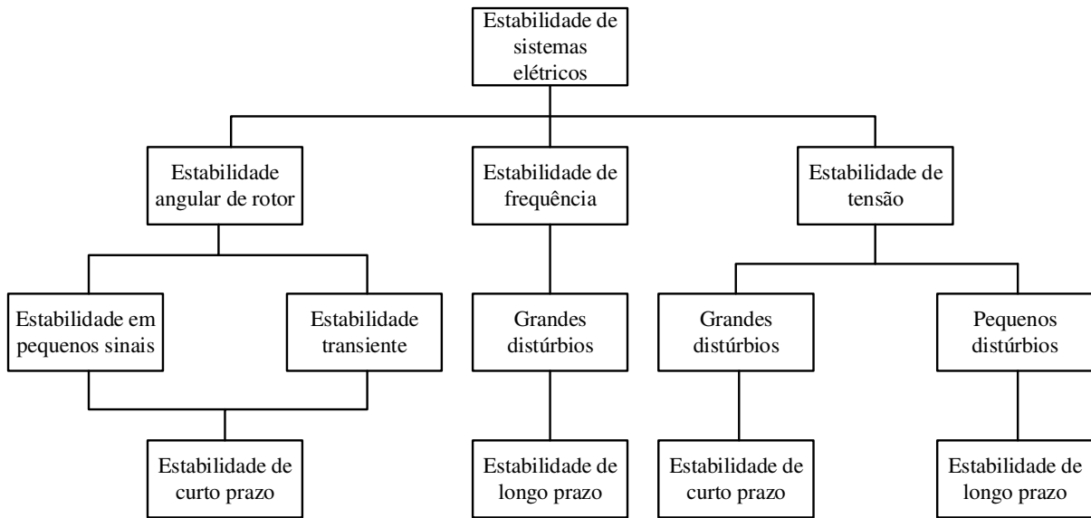
Figura 5 - Classificação da estabilidade em SEP
