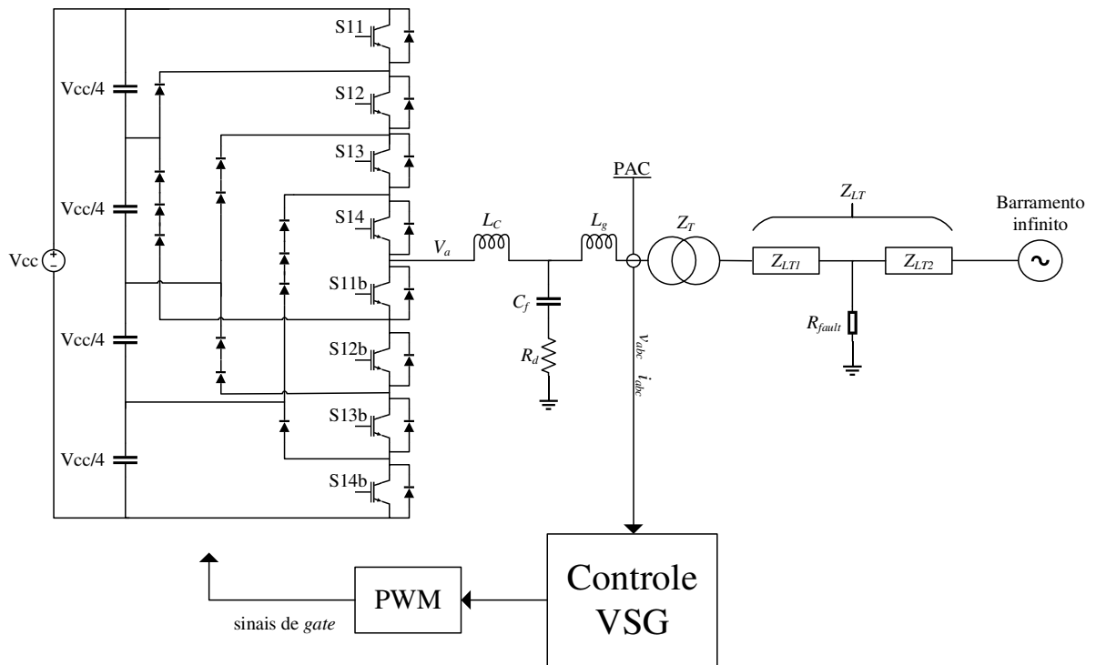
Figura 11 - Representação monofásica do sistema para simulação.
