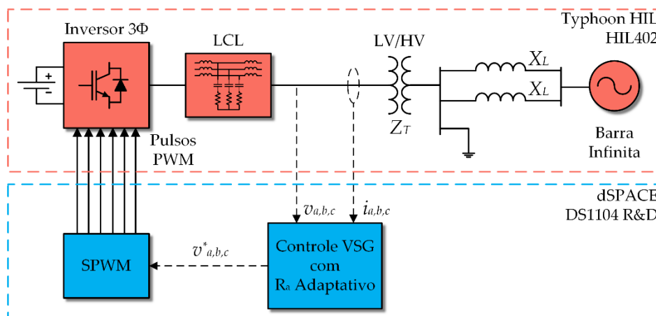
Figura 17 - Esquemático da bancada de testes em HIL.
