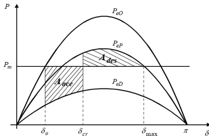
Gráfico 1 - Curvas de potência x ângulo para o sistema.
