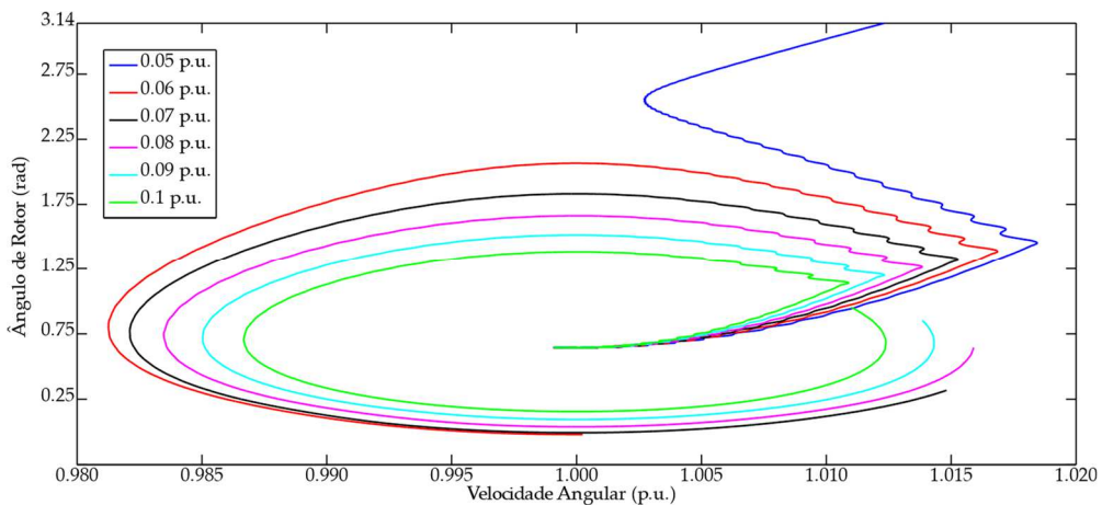
Gráfico 19 - Representação em plano de fase para um tempo de extinção de falta de 250 ms e diferentes valores de R_{SFCL} .
