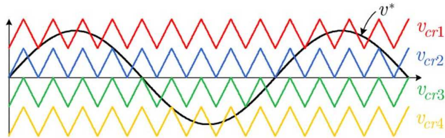
Figura 10 - Estratégia de chaveamento PWM do tipo PD.
