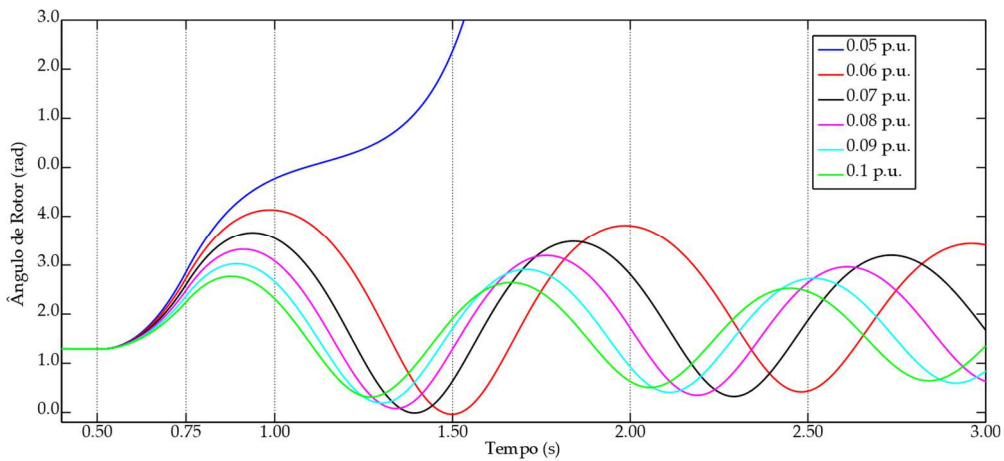
Gráfico 18 - Ângulo de rotor para um tempo de extinção de falta de 250 ms e diferentes valores de R_{SFCL} .
