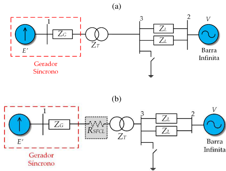
Figura 16 - Sistema SMIB para análise teórica: (a) sem resistência de SFCL; (b) com resistência de SFCL.
