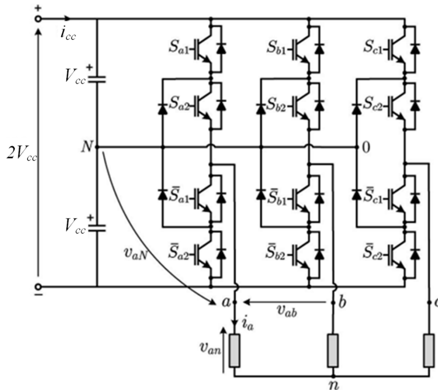
Figura 9 - Topologia clássica de um conversor NPC de 3 níveis.
