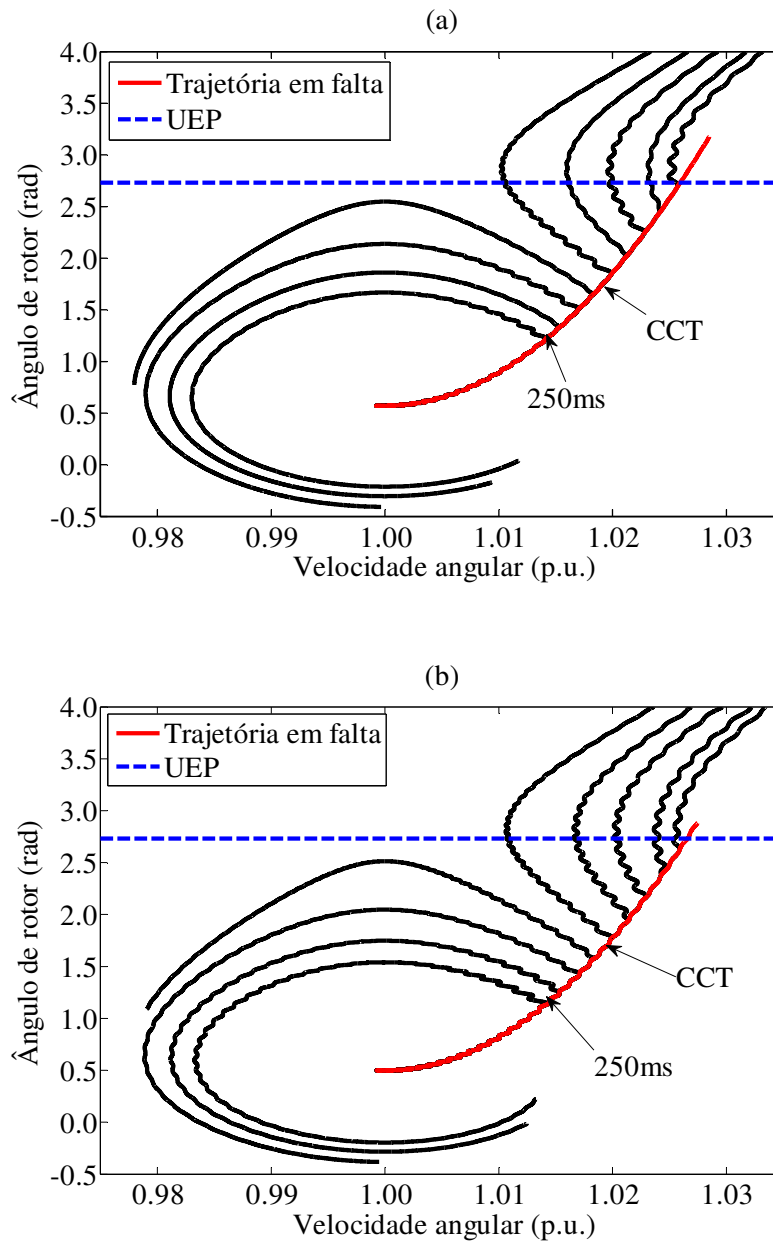
Gráfico 5 - Trajetórias do sistema com MS (a) e VSG (b) no plano de fase para o Cenário 6 e diferentes valores de t_{cl} .
