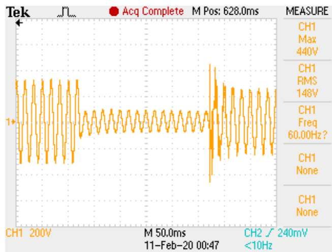
Figura 22 - Tensão de saída do VSG para um curto circuito com duração de 250 ms e R_{SFCL} = 0.10 p.u.
