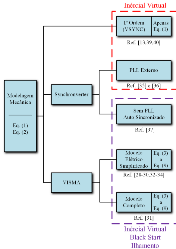
Figura 4 - Resumo das principais topologias de aplicação de máquinas síncronas virtuais.
