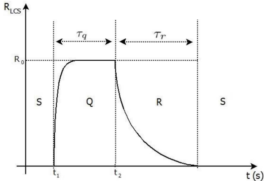
Gráfico 13 - Curva característica da resistência do SFCL.
