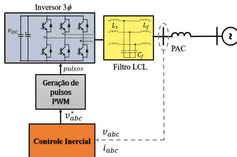
Figura 1 - Esquemático de controle para implementação de um VSG.
