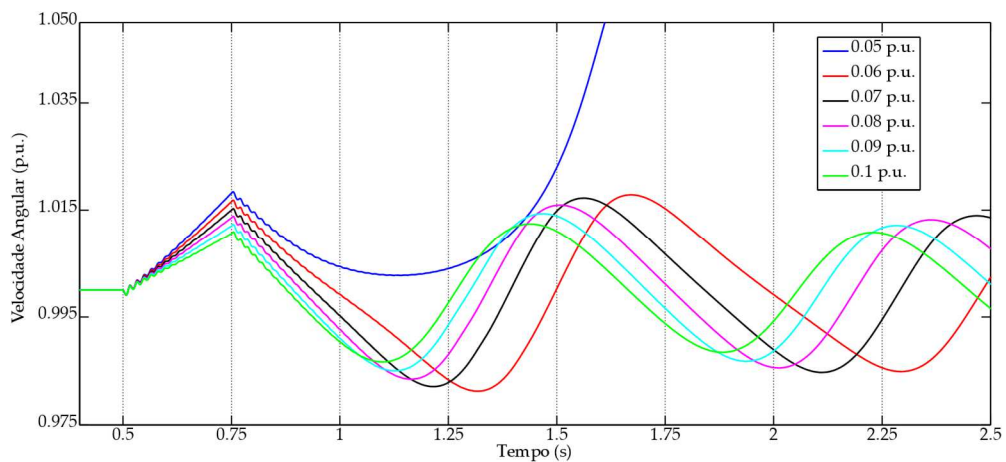
Gráfico 17 - Velocidade angular para um tempo de extinção de falta de 250 ms e diferentes valores de R_{SFCL} .
