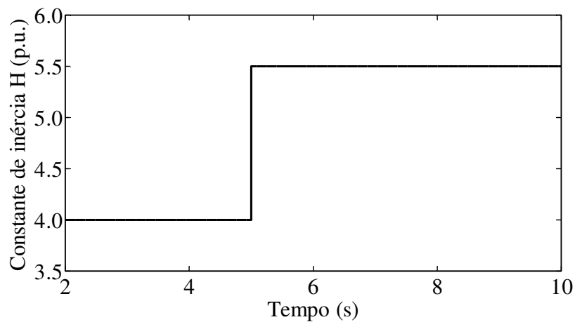
Gráfico 11 - Atuação do controle adaptativo no valor da constante de inércia H do VSG.
