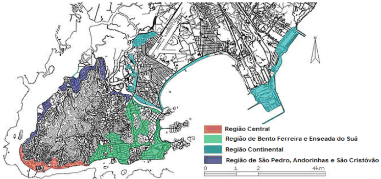
Figura 2 Aterros realizados em Vitória entre 1895 e 2000 (Marinato, 2004)
