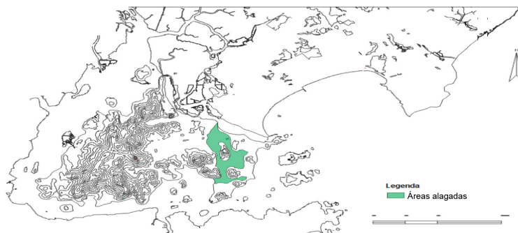
Figura 1 Vitória, excluindo-se as áreas de aterro nos limites das terras firmes da ilha - 1899 (MARINATO, 2004).
