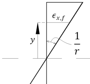
Figura 4.3 – Deformações de flexão na seção transversal
