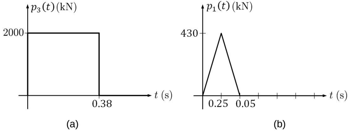
Figura 6.12 – Carregamentos atuantes nos sistemas Shear Buildings
