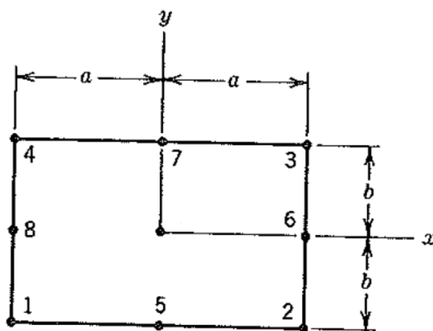
Figura 4.1 – Elemento quadrilateral quadrático de 8 nós
