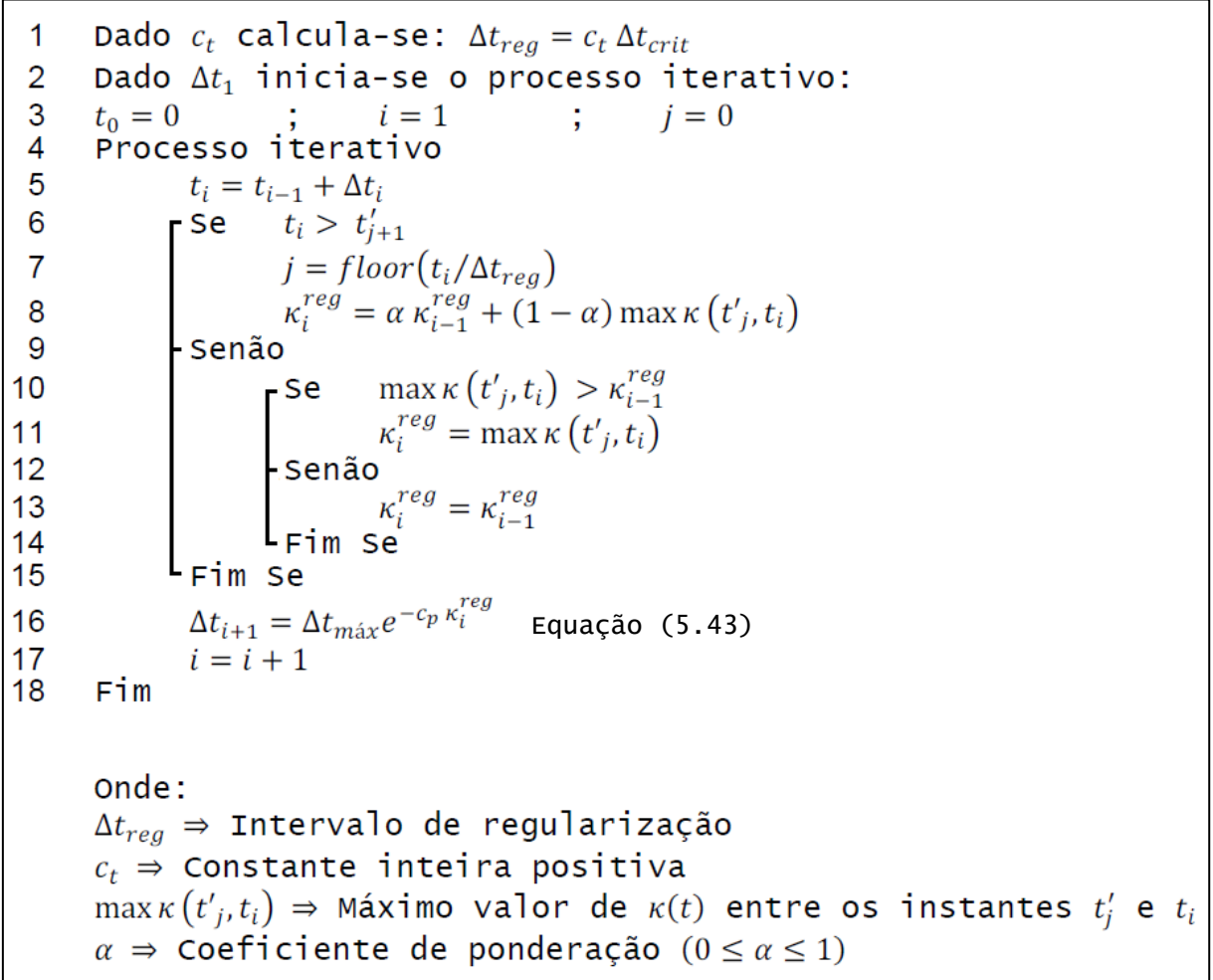
Figura 5.5 – Algoritmo de regularização por máximo valor em intervalos
