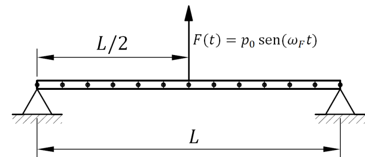
Figura 6.19 – Modelo de viga simplesmente apoiada sob carga senoidal
