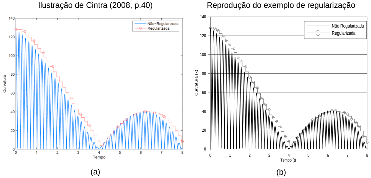
Figura 5.6 – Regularização de curvatura por máximo valor em intervalos
