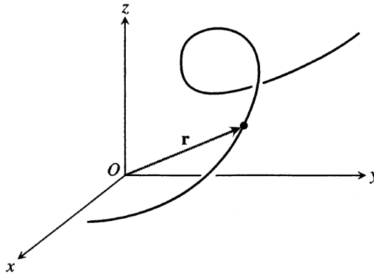
Figura 5.3 – Representação de uma curva paramétrica no espaço
