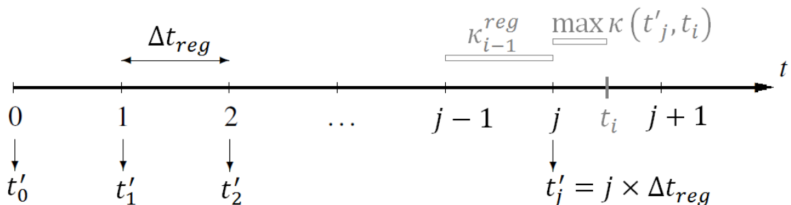
Figura 5.4 – Intervalos de regularização da curvatura
