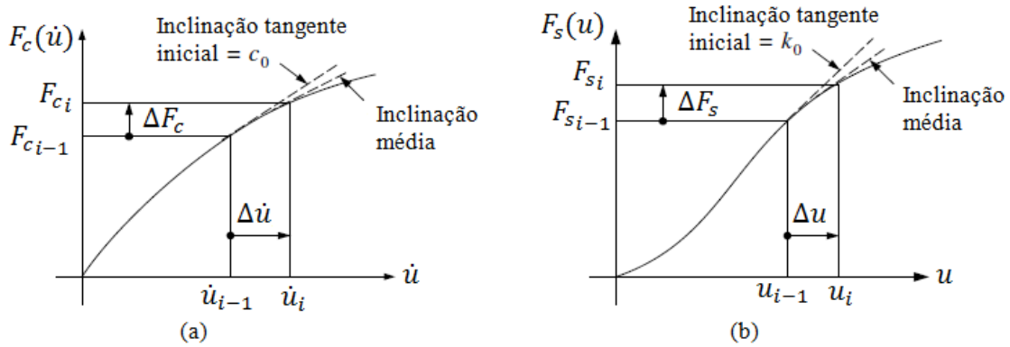
Figura 2.9 – Forças do sistema dinâmico não linear
