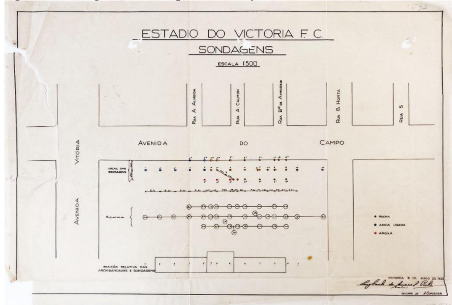
Figura 2. Sondagem realizada para construção do estádio do Victoria F. C. 1933.
