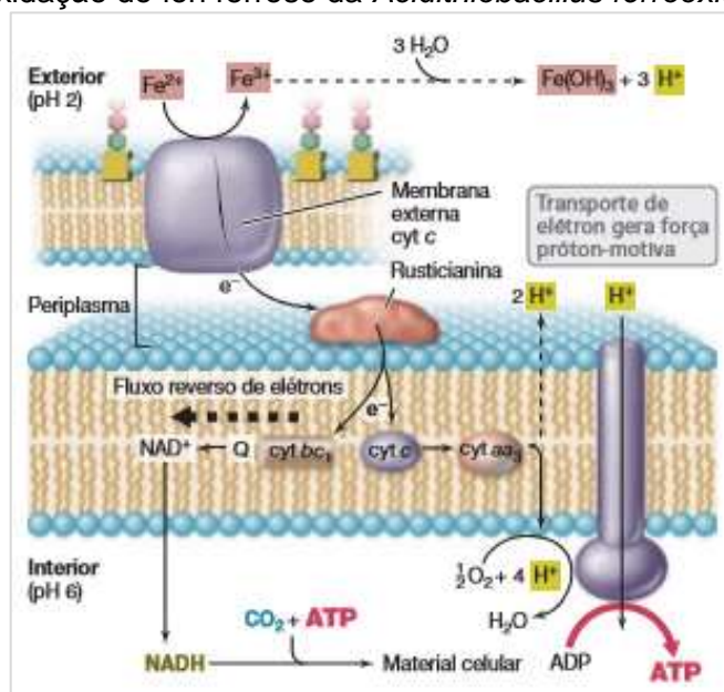
Figura 1- Esquema da geração de energia a partir da oxidação do íon ferroso da Acidithiobacillus ferrooxidans
