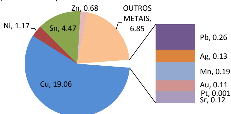
Figura 14 - Composição metálica das placas de circuito impresso de tablets (% em massa)
