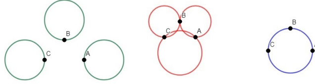
Figura 2.1: As circunferências em verde contém os subconjuntos unitários, as vermelhas contém os subconjuntos com dois pontos e a circunferência azul contém os três pontos.
