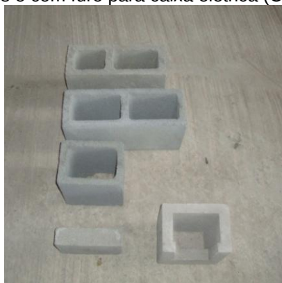
Figura 21 – Utilização de diferentes tamanhos de blocos e com furo para caixa elétrica (C.O.-1)
