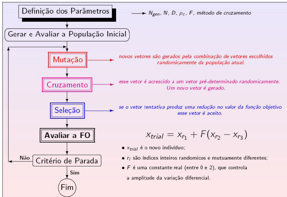
Figura 14- Esquema da aplicação do algoritmo de Evolução Diferencial.
