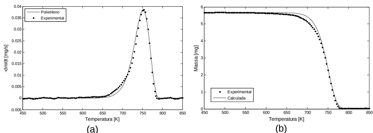
Figura 23- Decomposição do polietileno de baixa densidade: (a) Curvas DTG experimental e simulada com o modelo de reação global; (b) Curvas de perda de massa experimental e simulada com o modelo, para \beta = 20 K/min.
