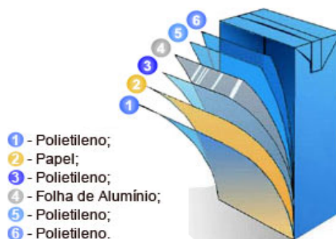
Figura 1- Estrutura da embalagem cartonada.
