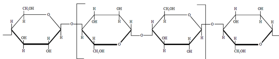
Figura 3- Estrutura química da celulose.
