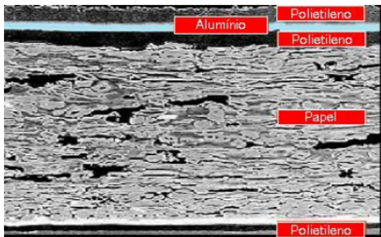
Figura 2- Corte transversal da embalagem cartonada mostrando as diferentes espessuras das suas multicamadas.
