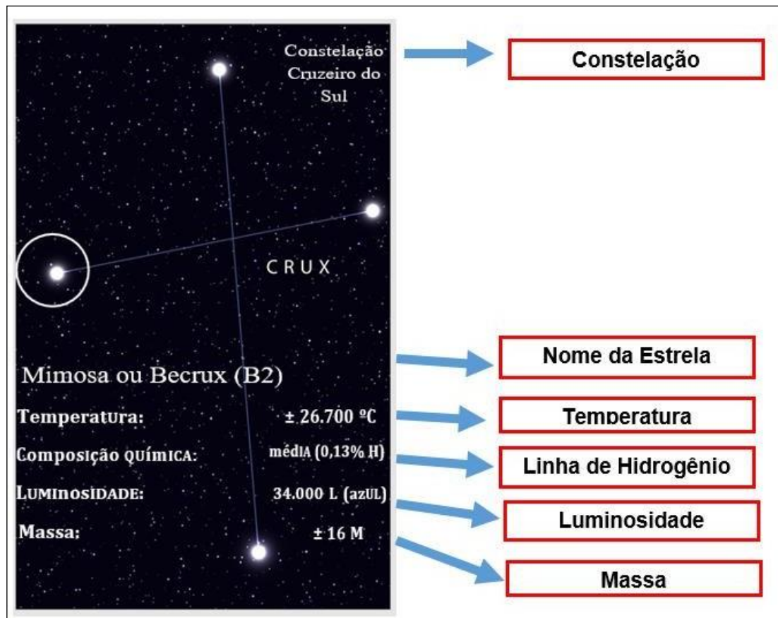
Figura 10a – Informações relativas à composição química das estrelas
