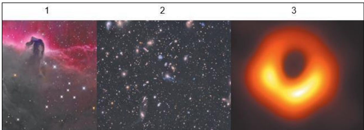
Figura 16 – O que existe no Universo?
