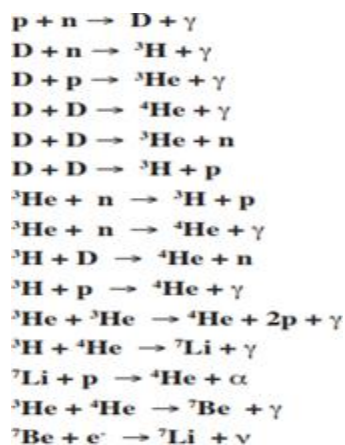
Figura 05 – Reações de Nucleossíntese
