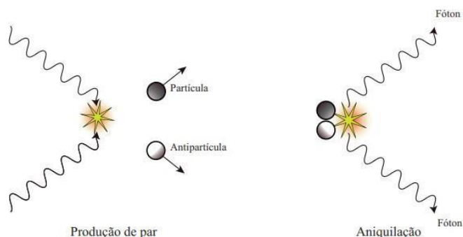
Figura 03 - Matéria e antimatéria: formação e aniquilação
