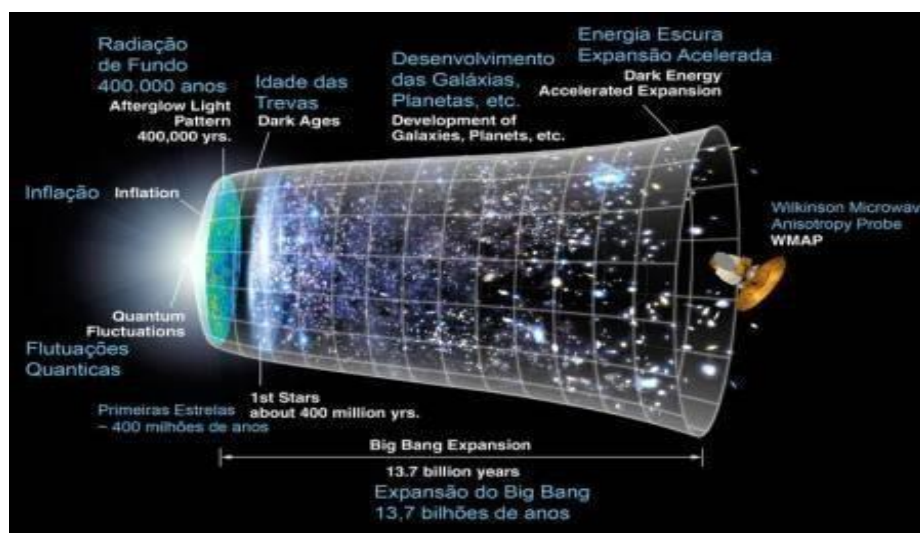
Figura 01: A evolução do Universo
