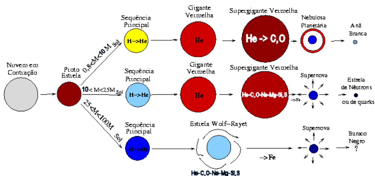
Figura 09 – Fases da Evolução Estelar
