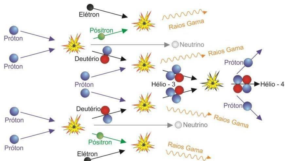
Figura 04 – Cadeia próton-próton
