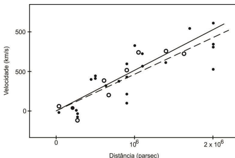
Figura 02: Diagrama de Hubble na forma original
