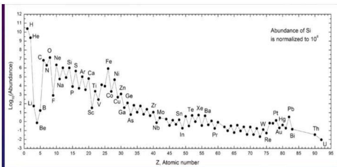
Figura 06 – Abundância relativa dos elementos
