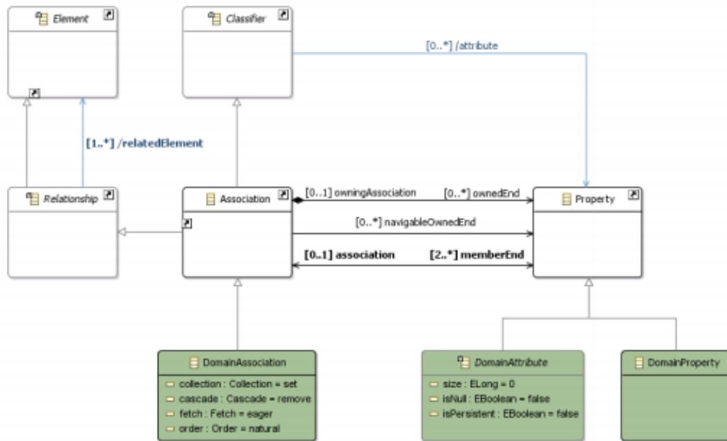
Figura 16 – Fragmento do metamodelo de Entidades: Associações (MARTINS, 2016)
