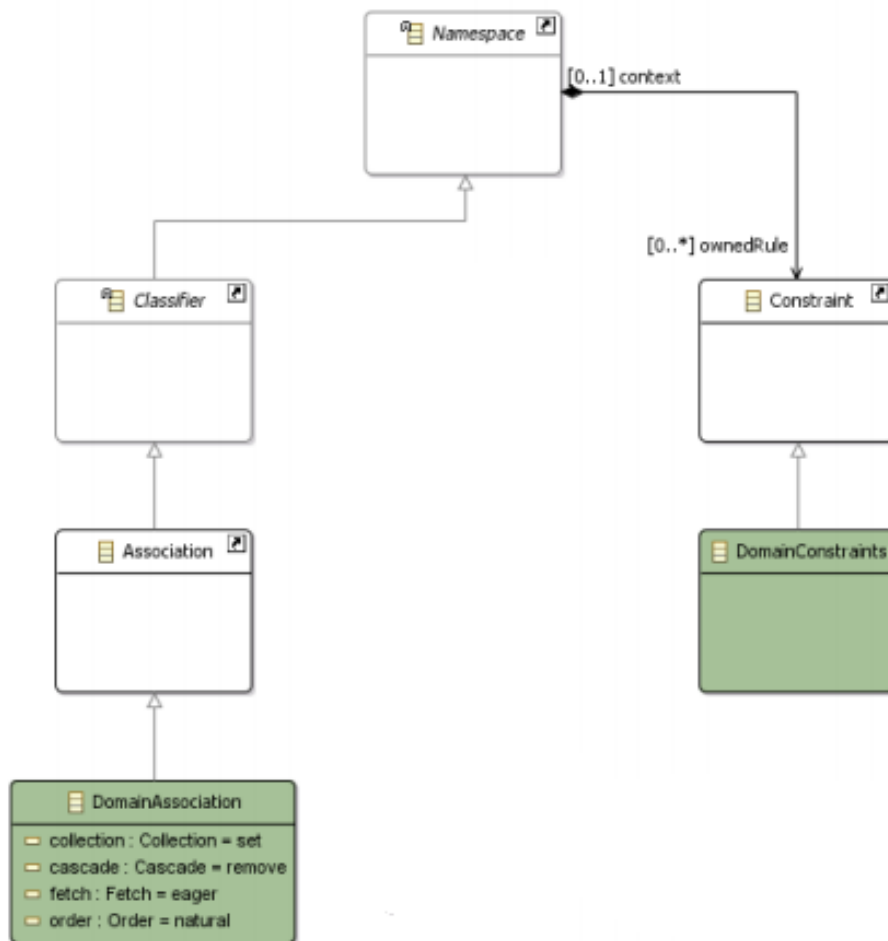
Figura 17 – Fragmento do metamodelo de Entidades: Restrições (MARTINS, 2016)
