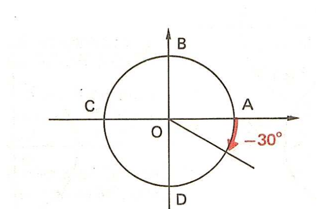
Figura 36: Arcos negativos
