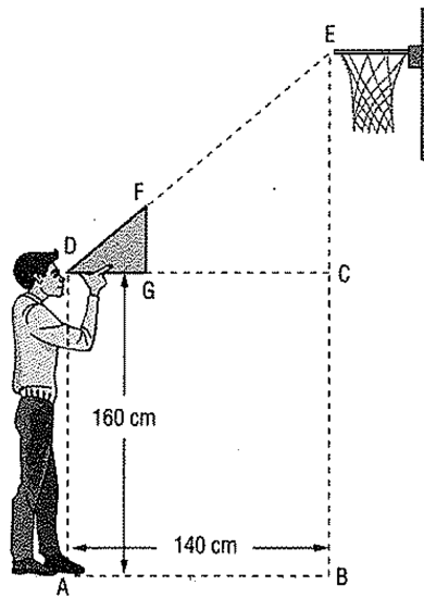
Figura 11: Problema da altura da cesta
