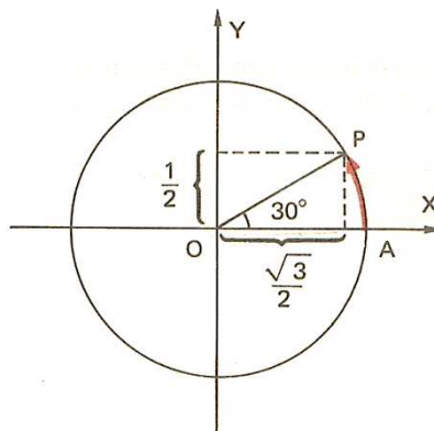
Figura 40: Abcissa e ordenada do arco de 30^\circ
