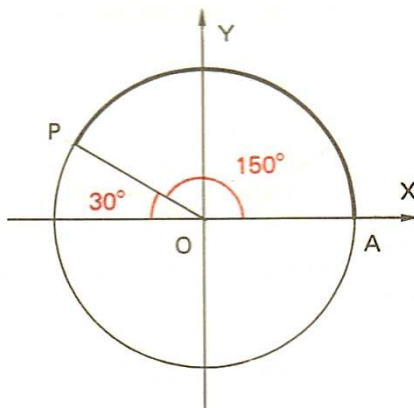
Figura 42: Arco de 150^\circ
