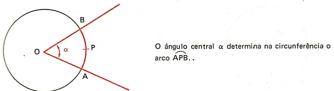
Figura 28: Ângulo central
