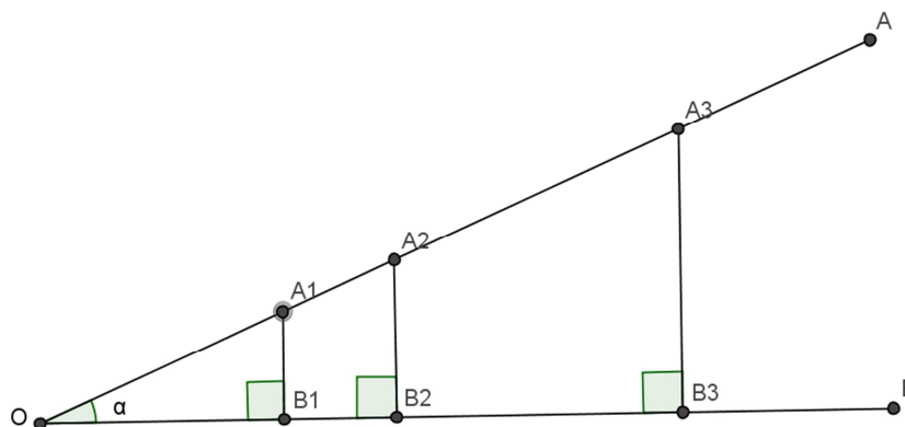
Figura 17: Funções trigonométricas
