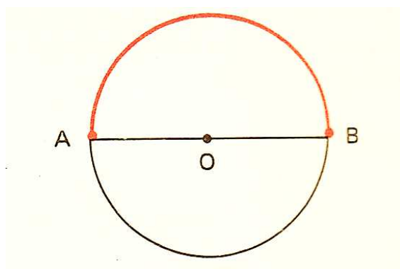
Figura 26: Semicircunferência
