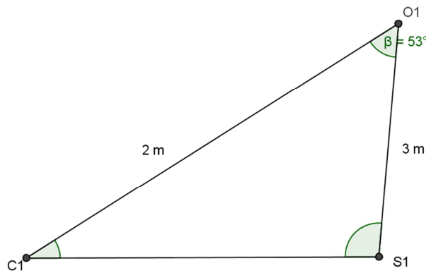
Figura 9: Triângulo O1C1S1
