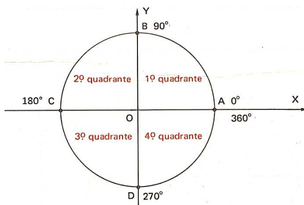
Figura 35: Quadrantes
