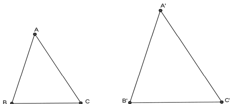
Figura 1: Semelhança de triângulos
