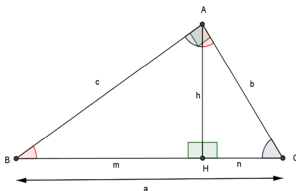
Figura 6: Relações métricas
