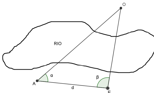
Figura 54: Problema da distância entre dois pontos
