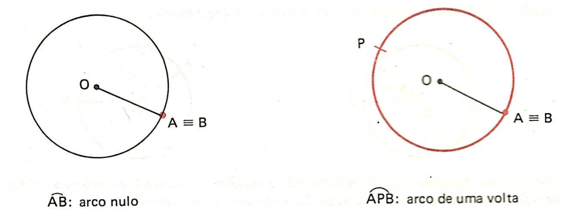
Figura 27: Arco nulo ou de meia volta
