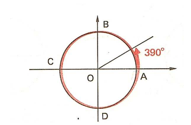
Figura 37: Arcos maiores que 360^\circ
