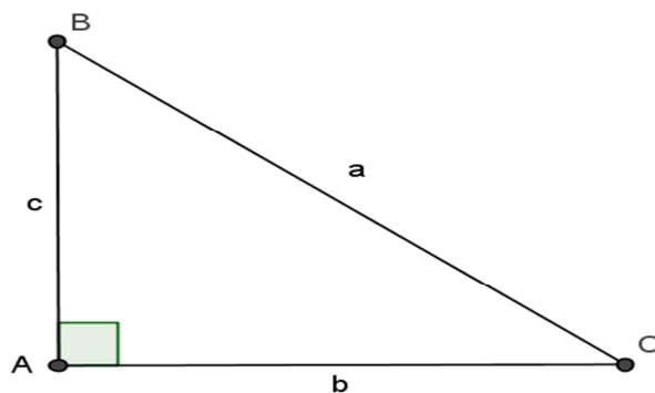
Figura 5: Triângulo retângulo
