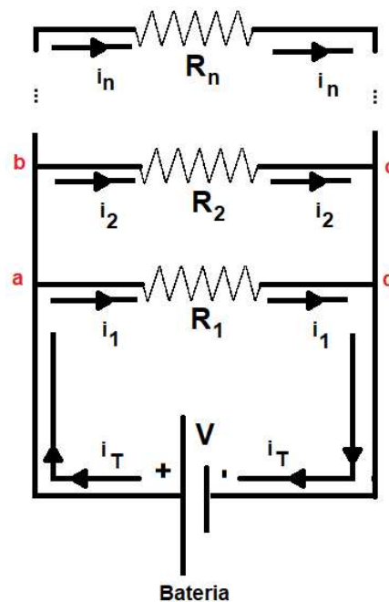
Figura 10 – Associação de resistores em paralelo
