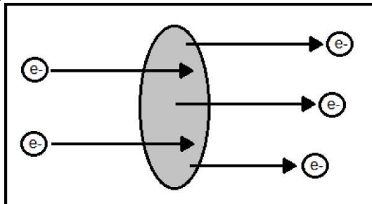
Figura 97- Cargas em movimento através de uma área A de um fio condutor.
