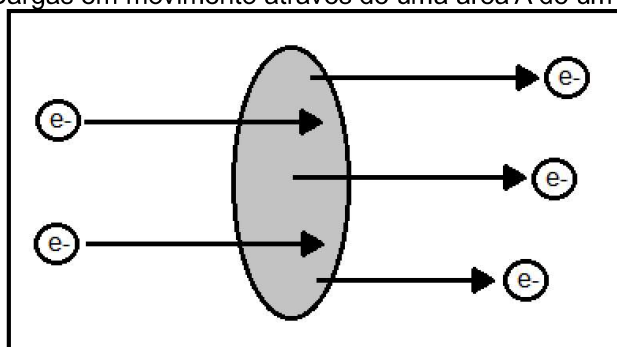
Figura 7- Cargas em movimento através de uma área A de um fio condutor.
