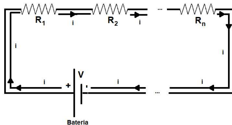
Figura 9 - Associação de resistores em série.
