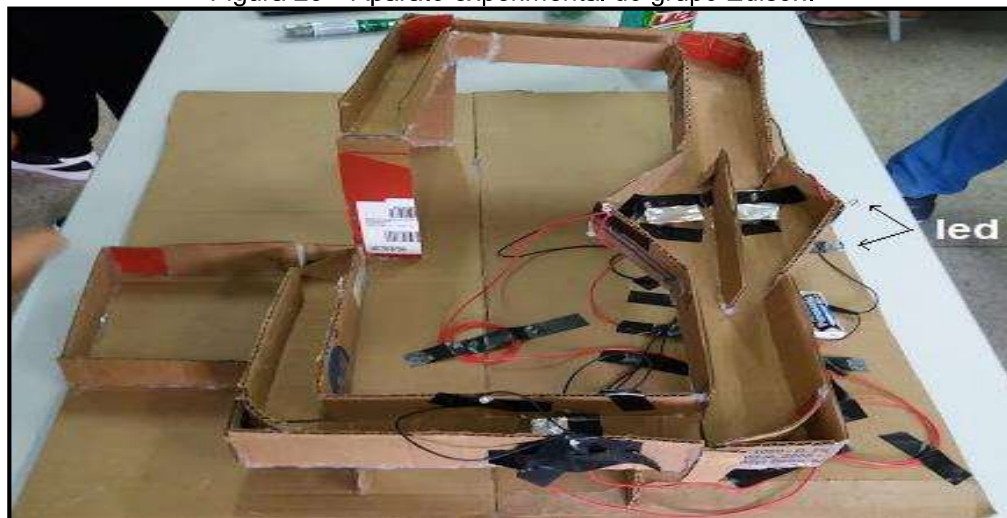
Figura 20 – Aparato experimental do grupo Edison.
