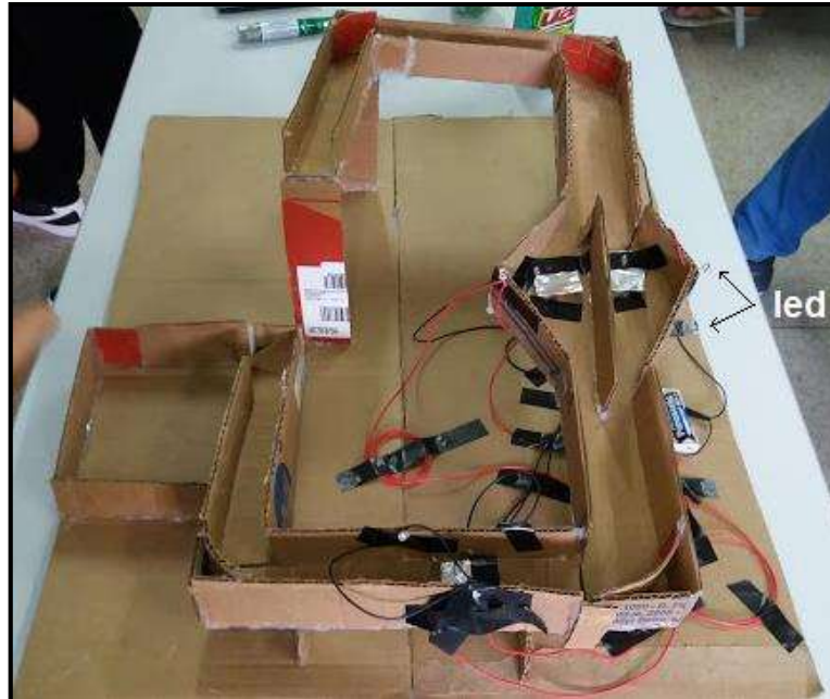
Figura 109 – Aparato experimental do grupo Edison.
