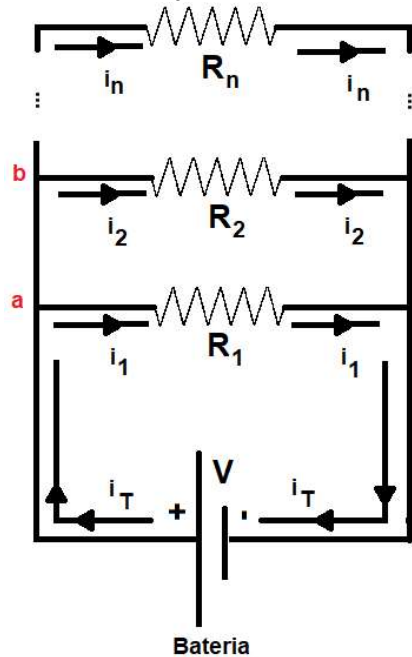
Figura 101 – Associação de resistores em paralelo
