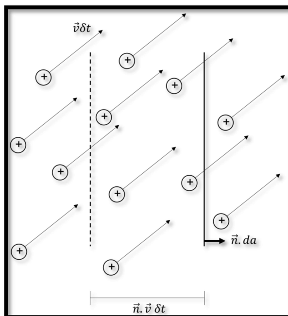
Figura 8 - Deslocamento dos portadores de cargas elétricas através do plano “ da ” no tempo \delta t .
