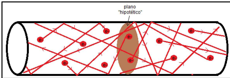
Figura 96 – Representação do movimento caótico dos elétrons de condução em um fio de cobre.
