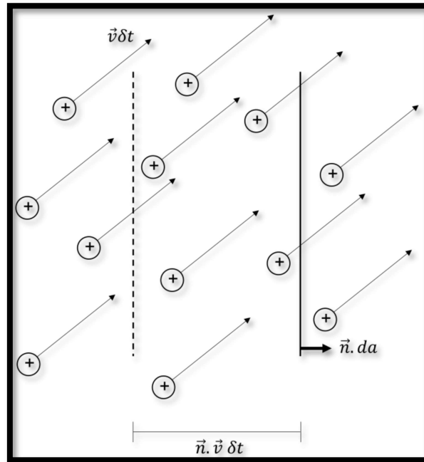
Figura 98 - Deslocamento dos portadores de cargas elétricas através do plano “da” no tempo \delta t .
