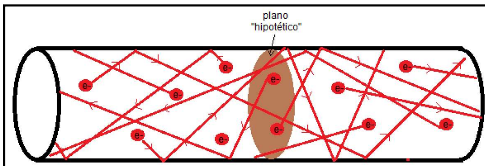
Figura 6 – Representação do movimento caótico dos elétrons de condução em um fio de cobre.
