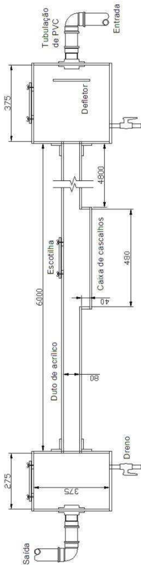
Figura 7 - Dimensões da montagem experimental (cotas em mm)
