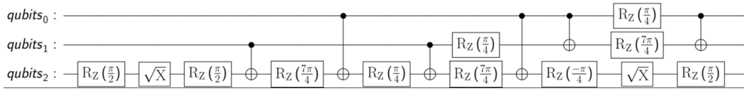
Figura 19 – Circuito quântico que realiza a porta Toffoli nos computadores quânticos da IBM.
