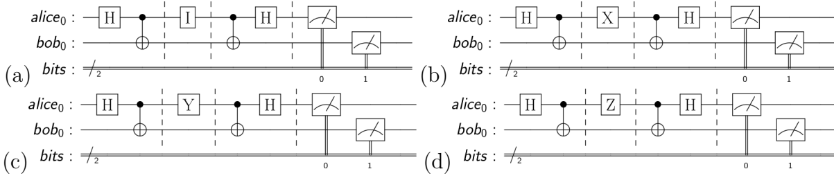
Figura 30 – Circuitos quânticos de codificação superdensa para a transmissão de dois bits clássicos.
