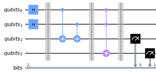
Figura 77 – Representação gráfica do circuito half-adder no formato matplotlib.
