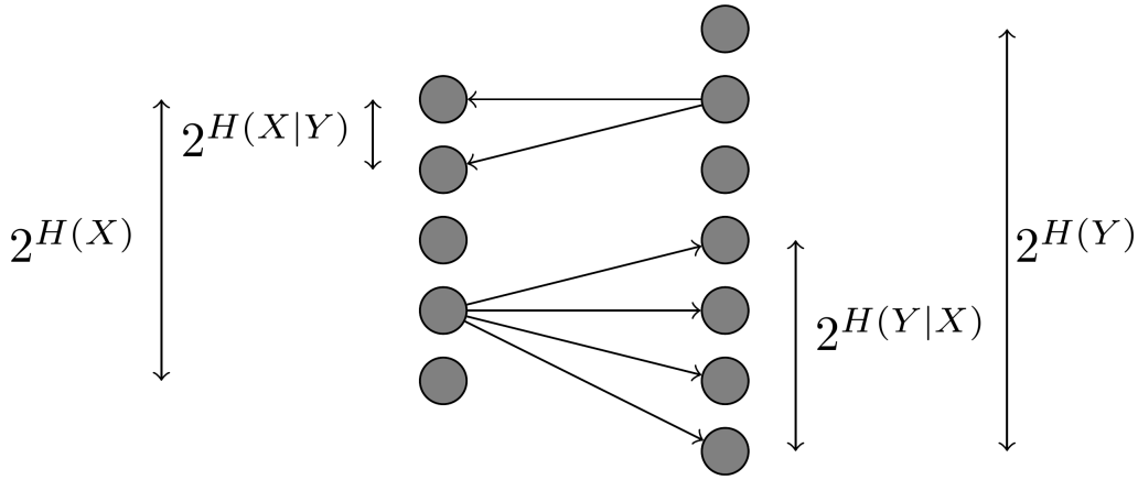
Figura 4 – Relação entre os sinais de entrada e os sinais de saída em um canal de transmissão com ruído.
