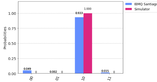
Figura 31 – Resultado de 8192 execuções do circuito quântico que transmite a mensagem 10 no simulador e na QPU ( Quantum Processor Unit ) IBMQ Santiago 5 qubits.
