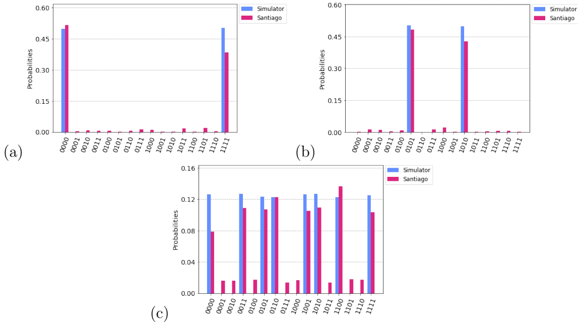
Figura 65 – Histogramas dos resultados de: (a) Preparação do estado (4.95); (b) Preparação do estado (4.96) e (c) Medição do estado (4.95) na base de estados de \sigma_x no computador quântico Santiago da IBM usando os circuitos (c) e (d) da Figura 63.
