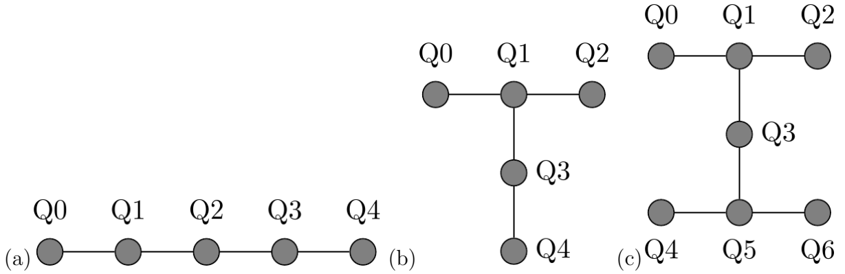
Figura 48 – Mapa de acoplamento dos qubits: (a) IBMQ Santiago; (b) IBMQ Belém e Lima e (c) IBMQ Lagos.
