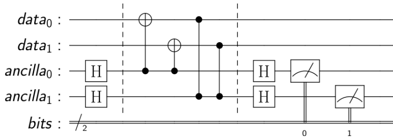
Figura 56 – Circuito que implementa o bloco fundamental dos surface codes .
