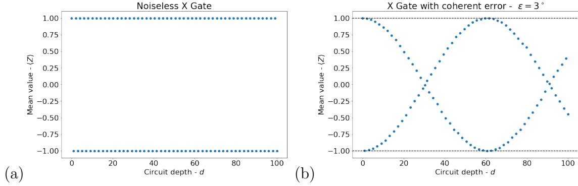
Figura 43 – Valor médio do operador Z para: (a) Estados da base computacional preparados por portas X perfeitas. (b) Estados da base computacional preparados por portas X com imperfeições causadas por erros coerentes que acrescentam \varepsilon = 3^\circ ao ângulo original da porta.
