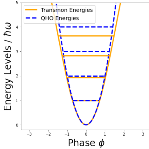
Figura 27 – Comparação entre os níveis de energia de um oscilador harmônico quântico e de um Transmon [43].
