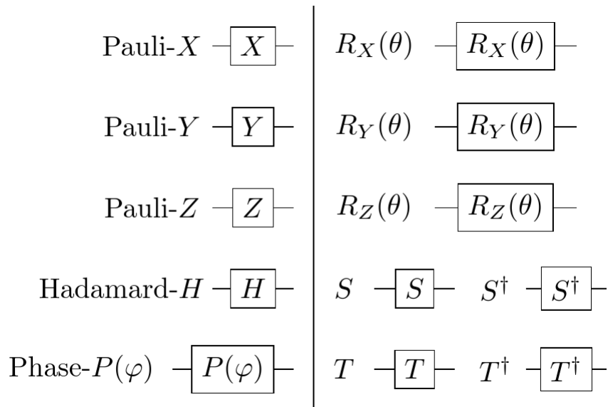
Figura 21 – Representações gráficas de algumas das portas que atuam sobre um qubit em um circuito quântico.
