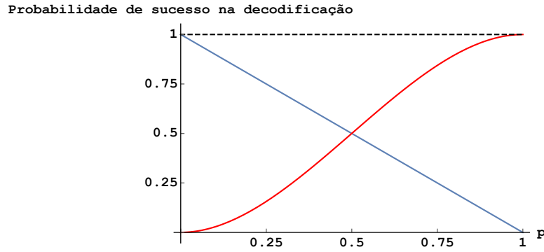
Figura 8 – Probabilidade de não ocorrer erro e de ocorrer erro em função da probabilidade de ocorrência de bit-flips .
