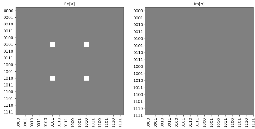
Figura 70 – Representação gráfica da matriz de densidade do estado de referência (4.96).
