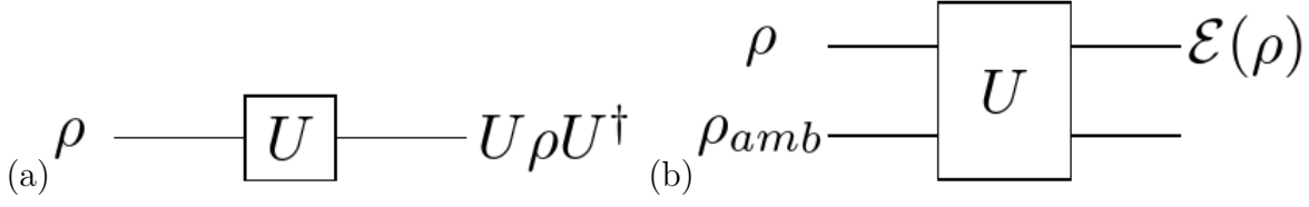
Figura 13 – (a) Modelo de evolução das matrizes densidade em sistemas quânticos fechados. (b) Modelo de evolução das matrizes de densidade em sistemas quânticos abertos.
