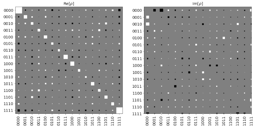
Figura 71 – Representação gráfica da matriz de densidade obtida através da tomografia de estado quântico realizada no circuito (c) da Figura 62.
