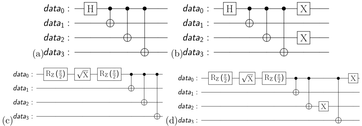
Figura 63 – Os circuitos (a) e (b) são uma versão alternativa dos circuitos apresentados em 62, já os circuitos (c) e (d) são as versões transpiladas que foram usadas nos experimentos realizados nos computadores Belém, Santiago e Lagos da IBM, cujos resultados são apresentados no texto.
