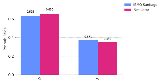
Figura 33 – Resultado de 8192 execuções do circuito quântico que realiza o teletransporte do estado |\psi\rangle = \sqrt{0.65}|0\rangle + \sqrt{0.35}|1\rangle no simulador e na QPU ( Quantum Processor Unit ) IBMQ Santiago 5 qubits.
