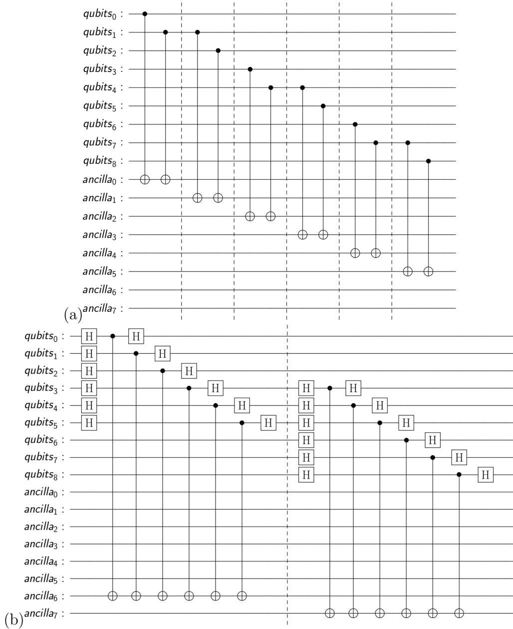
Figura 54 – Circuitos que executam as síndromes definidas pelo conjunto de estabilizadores \mathcal{S}_{[[9,1,3]]} .
