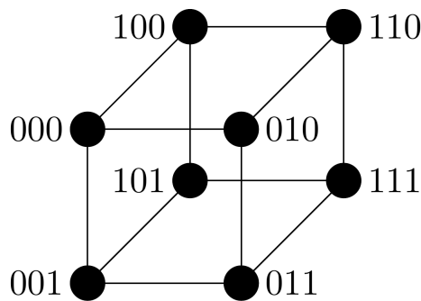
Figura 7 – Representação gráfica do código de repetição com distância d = 3 .
