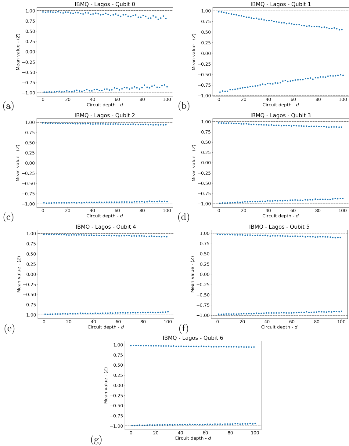
Figura 47 – Resultados do valor médio do operador Z calculado através da preparação dos estados na base computacional no computador quântico Lagos da IBM para os qubits: (a) Qubit 0; (b) Qubit 1; (c) Qubit 2; (d) Qubit 3; (e) Qubit 4; (f) Qubit 5 e (g) Qubit 6.
