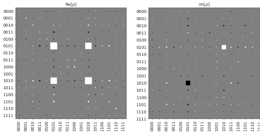
Figura 74 – Representação gráfica da matriz de densidade obtida através da tomografia de estado quântico realizada no circuito (d) da Figura 63.
