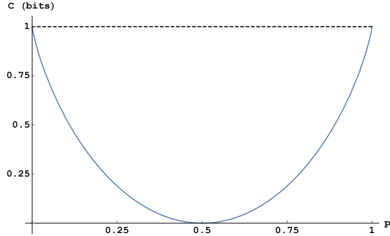
Figura 6 – Capacidade do canal binário simétrico.
