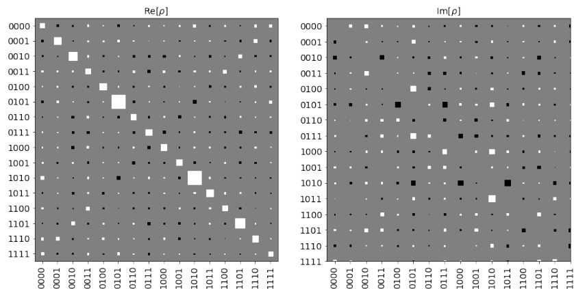
Figura 72 – Representação gráfica da matriz de densidade obtida através da tomografia de estado quântico realizada no circuito (d) da Figura 62.
