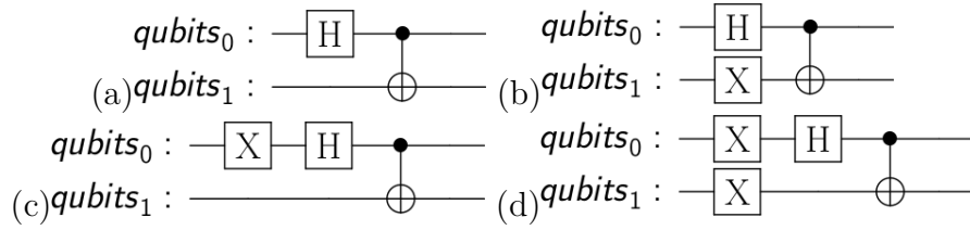
Figura 28 – Circuitos quânticos para criar os estados emaranhados: (a) |\psi_+\rangle (2.180); (b) |\phi_+\rangle (2.181); (c) |\psi_-\rangle (2.182) e (d) |\phi_-\rangle (2.183).
