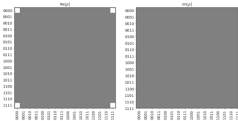
Figura 69 – Representação gráfica da matriz de densidade do estado de referência (4.95).
