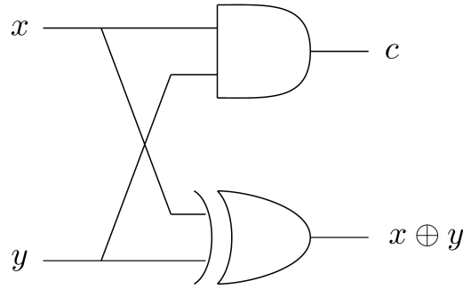
Figura 11 – Representação gráfica do circuito half-adder .
