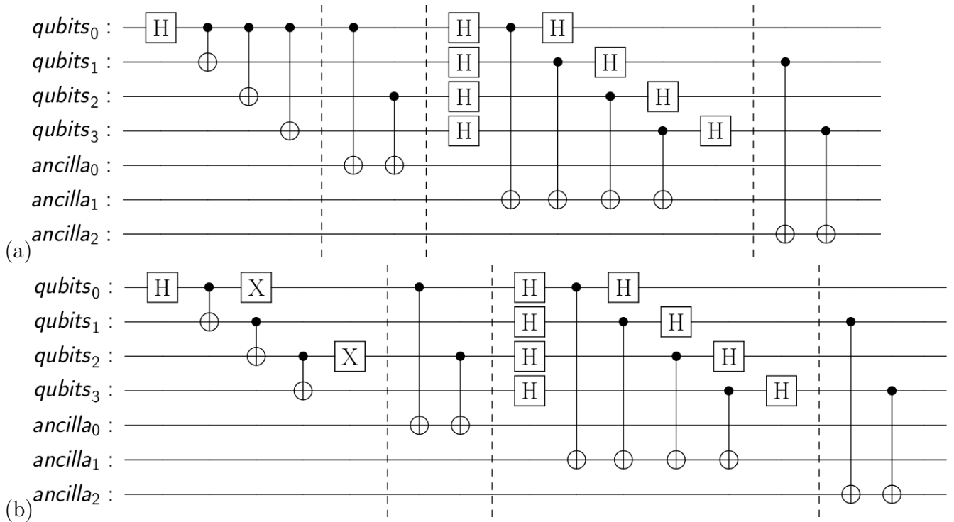
Figura 64 – Os circuitos (a) e (b) são uma versão alternativa dos circuitos apresentados em 62.
