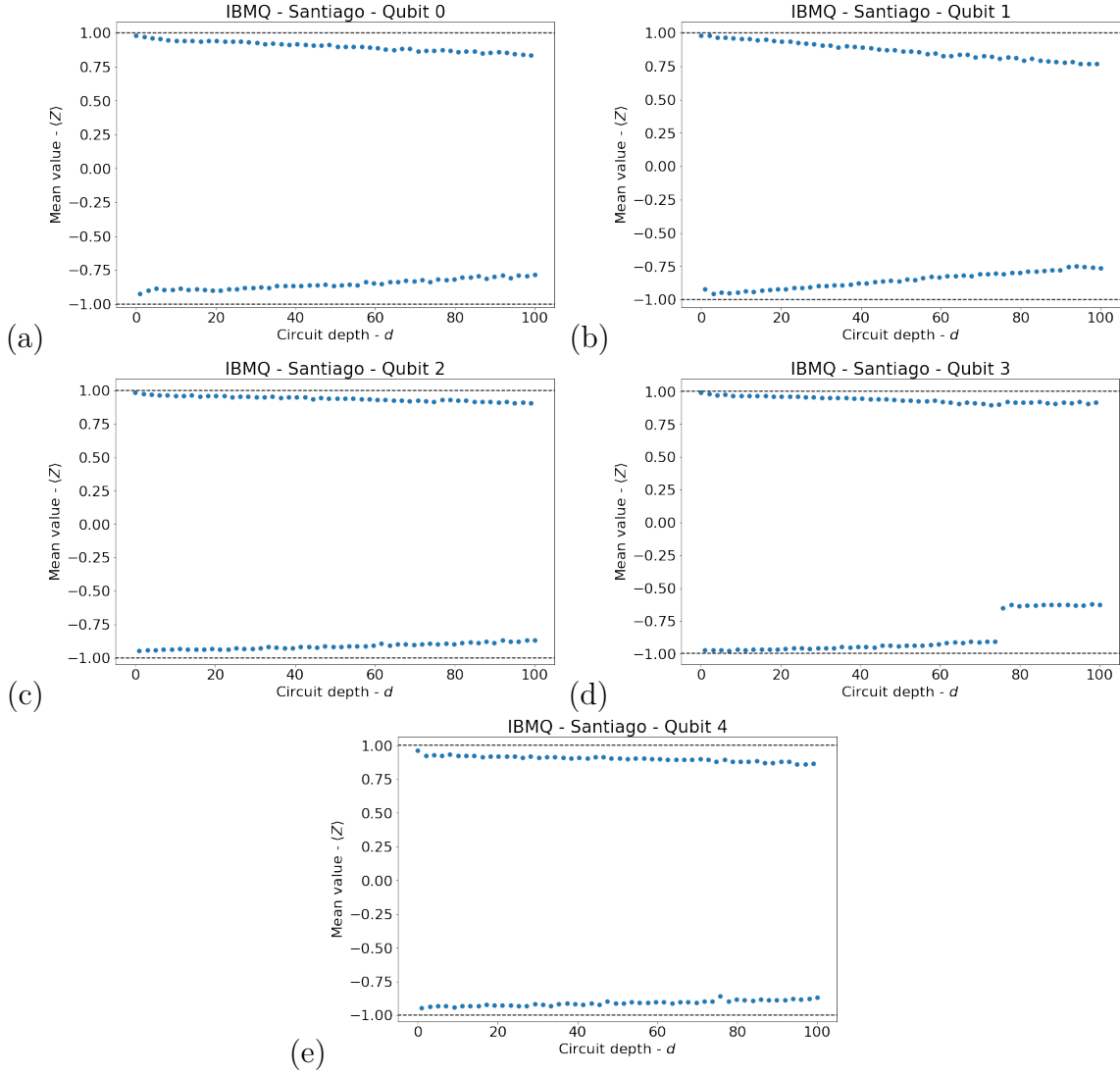
Figura 45 – Resultados do valor médio do operador Z calculado através da preparação dos estados na base computacional no computador quântico Santiago da IBM para os qubits: (a) Qubit 0; (b) Qubit 1; (c) Qubit 2; (d) Qubit 3 e (e) Qubit 4.
