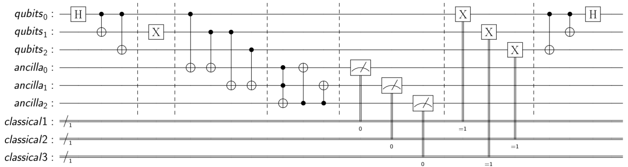
Figura 50 – Circuito quântico que representa a implementação do código [[3,1,3]] para corrigir um único bit-flip .
