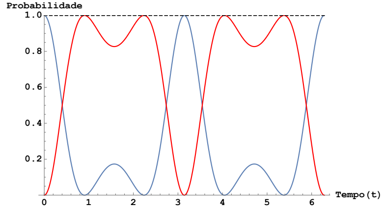
Figura 26 – Probabilidade de se medir os estados |0\rangle (curva azul) e |1\rangle (curva vermelha) em um instante de tempo t dado os parâmetros \gamma B_0 = 1 , \omega = 4 e n = 1 .
