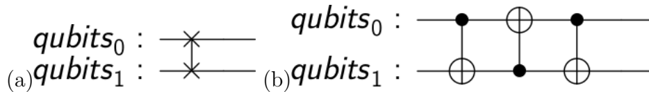
Figura 18 – Representações gráficas da porta SWAP: (a) convencional e (b) alternativa.
