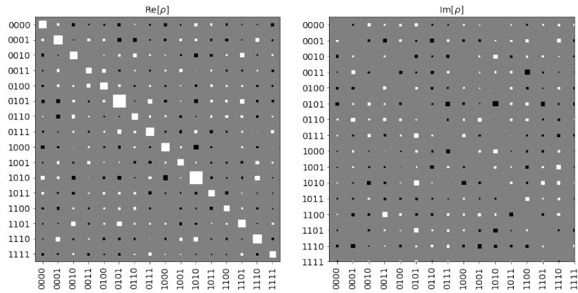
Figura 76 – Representação gráfica da matriz de densidade obtida através da tomografia de estado quântico realizada no circuito (b) da Figura 64.
