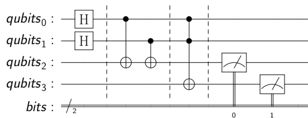
Figura 79 – Representação gráfica do circuito half-adder no formato LaTeX.
