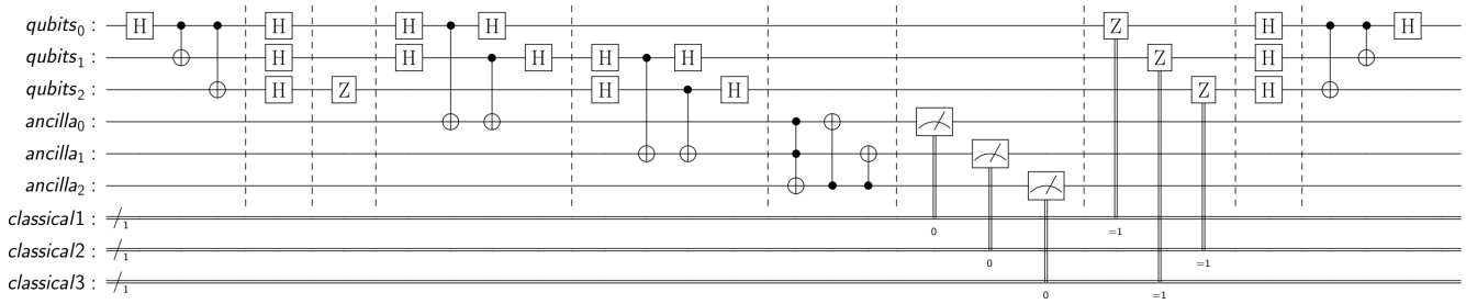
Figura 51 – Circuito quântico que representa a implementação do código [[3,1,3]] para corrigir um único phase-flip .
