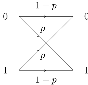
Figura 5 – Canal binário simétrico com probabilidade p de ocorrência de um bit-flip . À esquerda temos a entrada do canal com as mensagens enviadas e à direita temos as mensagens recebidas no final do canal.
