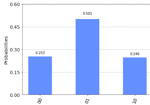
Figura 80 – Histograma representando o resultado obtido após a execução do circuito de half-adder com as entradas em superposição.
