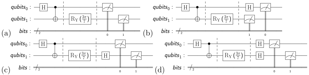
Figura 34 – Alguns dos circuitos quânticos utilizados para demonstrar a violação da desigualdade de Bell nos computadores quânticos Santiago, Belém e Lagos da IBM. No início de cada circuito é preparado o estado emaranhado (2.180), onde o qubit 0 representa o qubit de Alice e o qubit 1 o de Bob. Após essa etapa temos a aplicação de uma porta R_Y no qubit de Bob para realizar a rotação entre as bases de medida escolhidas por Alice e Bob. Nos circuitos presentes em (b), (c) e (d) temos a aplicação de portas Hadamard antes da medição, isso é feito para mudar a base de medição para os autoestados de \sigma_x , pois neste cenário Alice e Bob podem escolher medir se vão realizar medidas em termos dos autoestados de \sigma_z e \sigma_x .
