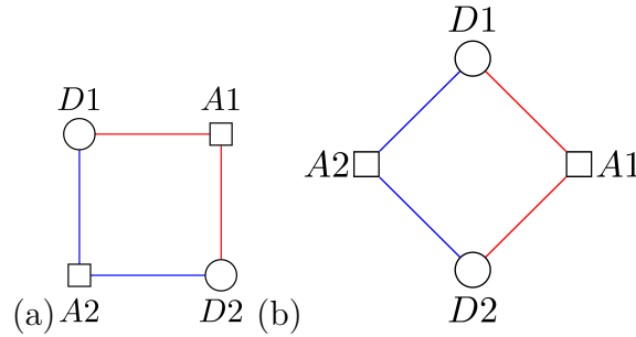
Figura 55 – Representações mais comuns do bloco fundamental dos surface codes .
