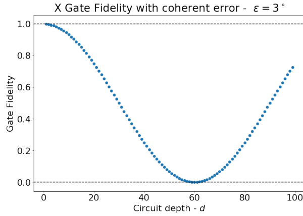
Figura 44 – Comportamento da fidelidade da porta X imperfeita de acordo com a profundidade do circuito.
