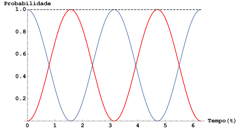
Figura 25 – Probabilidade de se medir os estados |0\rangle (curva azul) e |1\rangle (curva vermelha) em um instante de tempo t dado os parâmetros \gamma B_0 = 2 e n = 1 .
