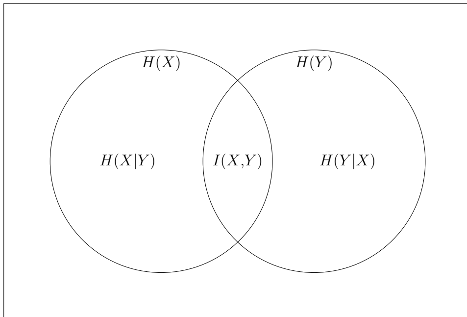
Figura 3 – Representação em diagrama de Venn da equação (1.34).
