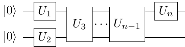
Figura 23 – Exemplo de uma sequência de aplicações de operadores que formam um circuito.
