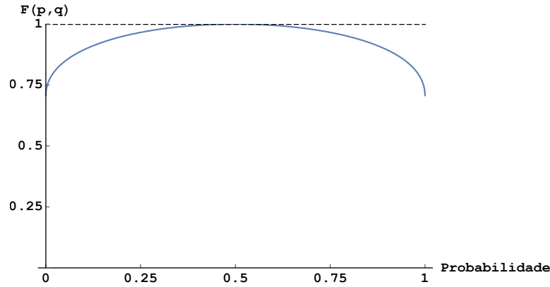
Figura 14 – Exemplo da fidelidade clássica entre as distribuições de probabilidade clássicas \{1/2, 1/2\} e \{p, 1 - p\} .
