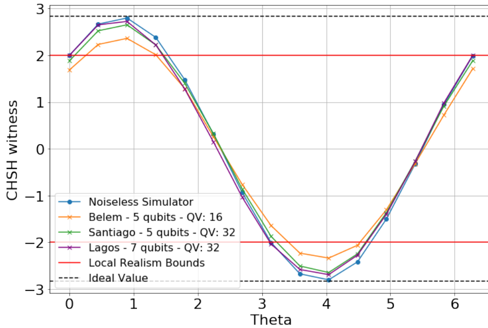
Figura 35 – Resultados das desigualdades CHSH para os computadores quânticos Santiago, Belém e Lagos da IBM.
