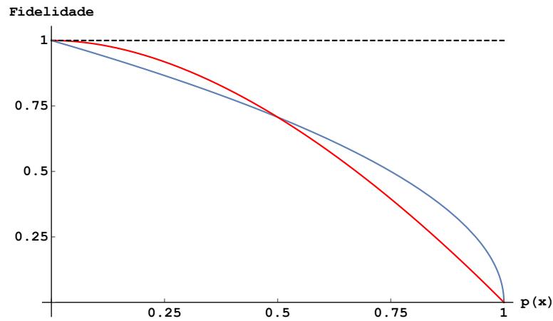
Figura 52 – Comparação dos comportamentos de F e F' em função da probabilidade de ocorrência de bit-flips .
