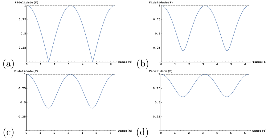
Figura 15 – Gráficos de (2.173) em função do tempo para diferentes valores de |a|^2 e |b|^2 . Aqui é possível ver que só ocorre transição entre os estados no cenário do primeiro gráfico. (a) |a|^2 = |b|^2 = 0.5 (b) |a|^2 = 0.6 e |b|^2 = 0.4 (c) |a|^2 = 0.7 e |b|^2 = 0.3 (d) |a|^2 = 0.8 e |b|^2 = 0.2 .
