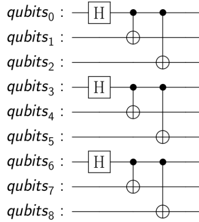
Figura 53 – Circuito de codificação do estado lógico |0_L\rangle_{Shor} .
