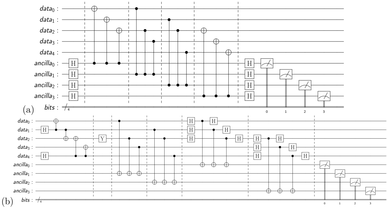
Figura 58 – Circuitos que implementam o surface code [[5,1,2]] : (a) Codificação pelo método de estabilizadores. (b) Codificação com portas do grupo de Clifford. O circuito na figura está detectando um erro Y no qubit D2 .
