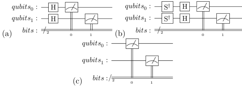
Figura 37 – Circuitos de medida nas bases: (a) X ; (b) Y e (c) Z .
