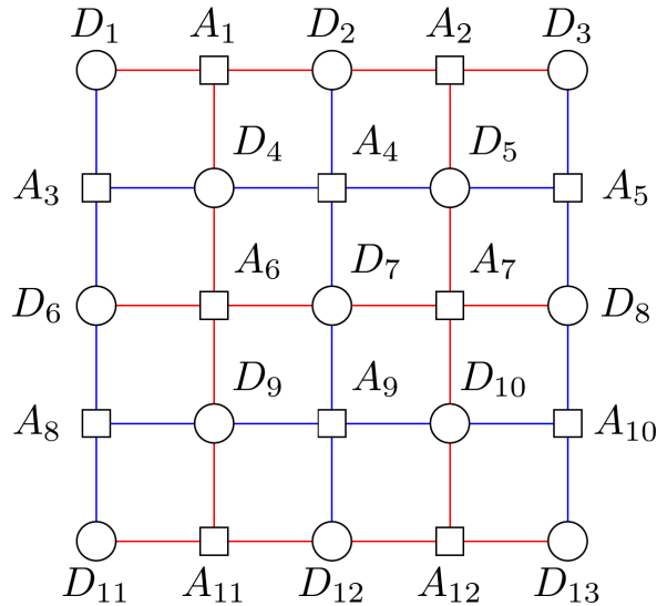
Figura 60 – Representação gráfica do surface code [[13,1,3]] .
