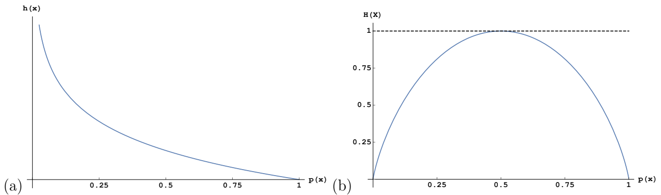
Figura 2 – (a) Comportamento da surpresa de acordo com a previsibilidade do resultado do evento. (b) Entropia Binária de Shannon.
