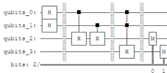
Figura 78 – Representação gráfica do circuito half-adder no formato texto.
