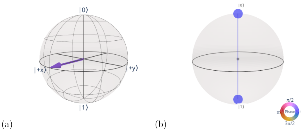
Figura 81 – (a) Exemplo de uma esfera de Bloch. (b) Exemplo de uma Qsphere.
