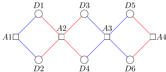
Figura 59 – Representação gráfica do surface code [[6,2,2]] .
