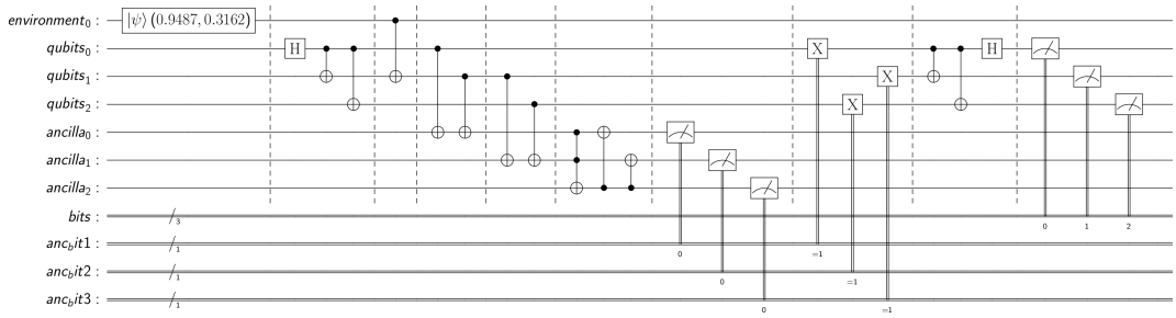
Figura 49 – Circuito que representa um canal de bit-flip onde a probabilidade de ocorrer este erro é p = 0.1 .
