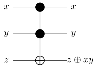
Figura 10 – Representação gráfica da porta Toffoli.
