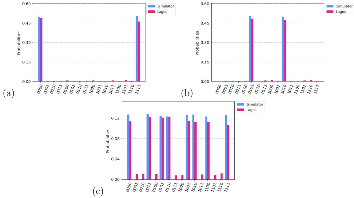
Figura 68 – Histogramas dos resultados de: (a) Preparação do estado (4.95); (b) Preparação do estado (4.96) e (c) Medição do estado (4.95) na base de estados de \sigma_x no computador quântico Lagos da IBM usando os circuitos (c) e (d) da Figura 63.
