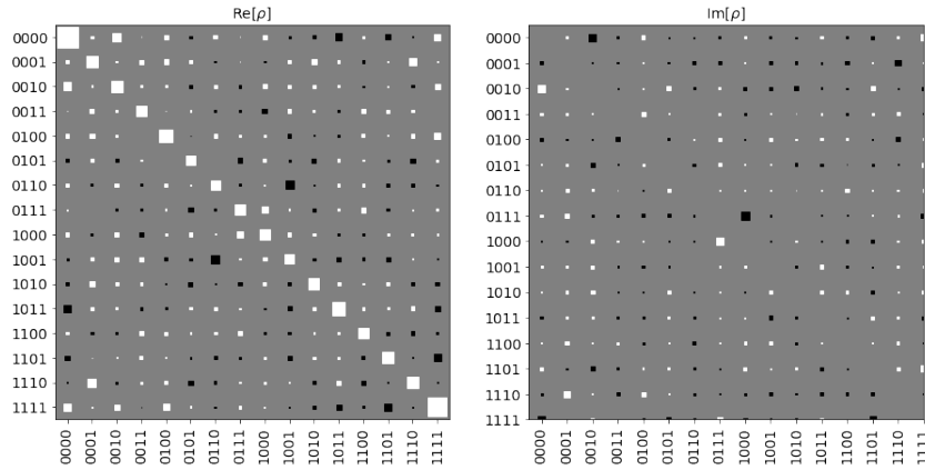
Figura 75 – Representação gráfica da matriz de densidade obtida através da tomografia de estado quântico realizada no circuito (a) da Figura 64.
