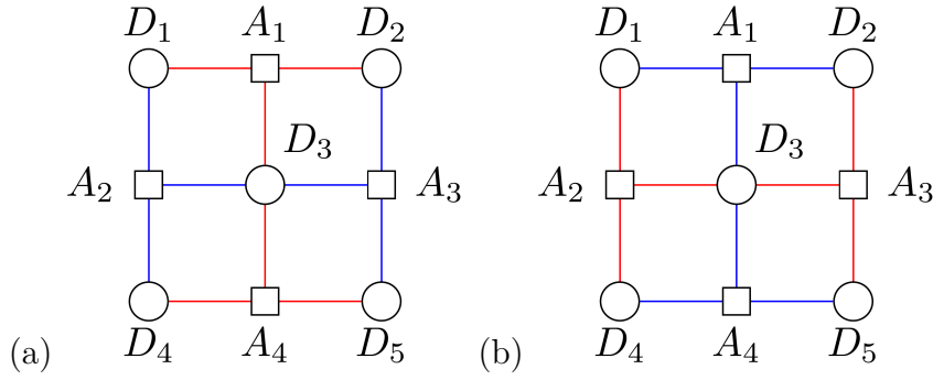
Figura 57 – Representação gráfica do surface code [[5,1,2]] . (a) Código original. (b) Código dual.
