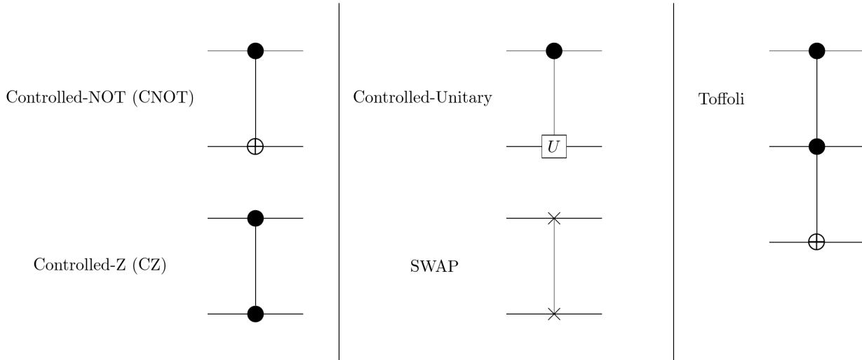
Figura 22 – Representações gráficas de algumas das portas de controle que aparecem em circuitos quânticos.
