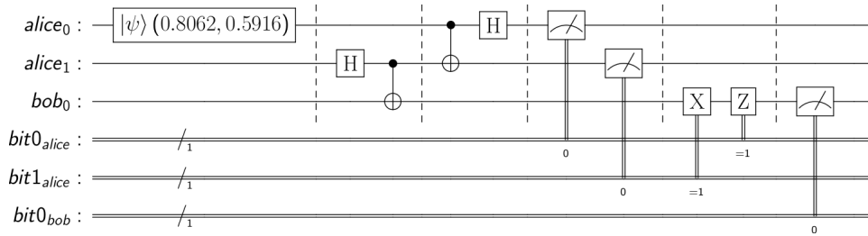
Figura 32 – Circuito quântico que executa um teletransporte quântico de um estado quântico |\psi\rangle .
