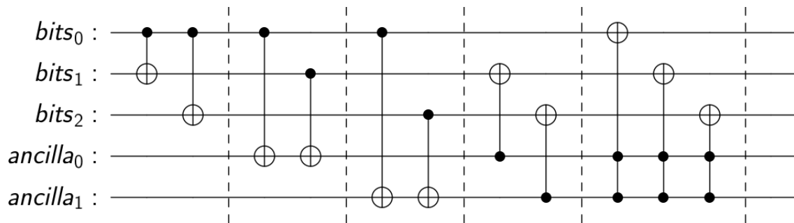
Figura 12 – Representação gráfica do circuito que realiza o código de repetição de 3 bits apresentado na seção anterior.
