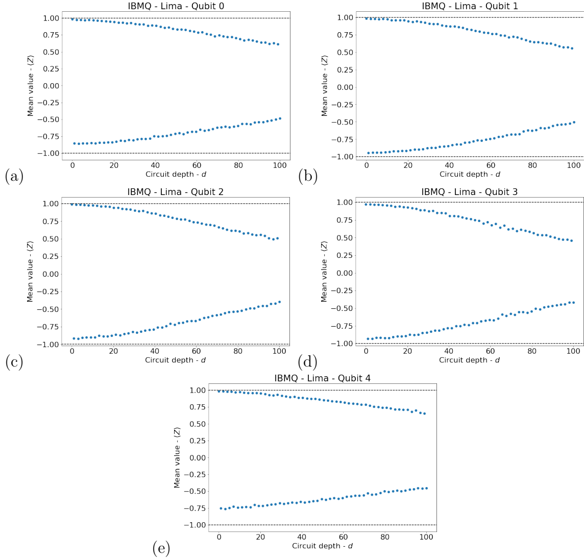
Figura 46 – Resultados do valor médio do operador Z calculado através da preparação dos estados na base computacional no computador quântico Lima da IBM para os qubits: (a) Qubit 0; (b) Qubit 1; (c) Qubit 2; (d) Qubit 3 e (e) Qubit 4.
