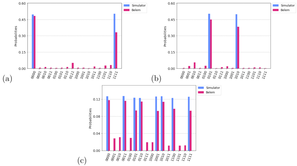
Figura 66 – Histogramas dos resultados de: (a) Preparação do estado (4.95); (b) Preparação do estado (4.96) e (c) Medição do estado (4.95) na base de estados de \sigma_x no computador quântico Belém da IBM usando os circuitos (c) e (d) da Figura 63.
