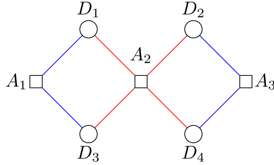
Figura 61 – Representação gráfica do mapa de acoplamento dos qubits usados nos experimentos conduzidos na referência [17] e do surface code [[4,1,2]] implementado no dispositivo.
