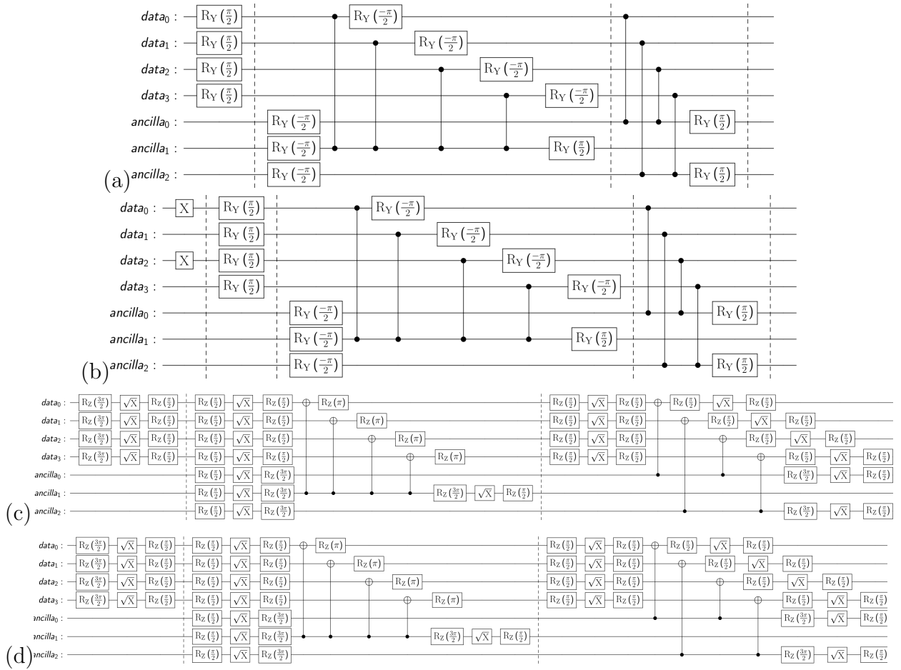
Figura 62 – Os circuitos (a) e (b) foram utilizados para realizar a codificação e síndrome do código [[4,1,2]] em [17]. Os circuitos (c) e (d) são as versões transpiladas que foram executados no computador Lagos da IBM para obter os dados discutidos no texto.
