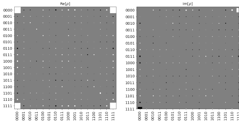
Figura 73 – Representação gráfica da matriz de densidade obtida através da tomografia de estado quântico realizada no circuito (c) da Figura 63.
