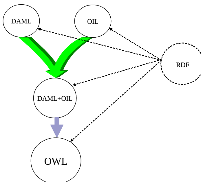
Figura 4.7 – Origem da Linguagem OWL
