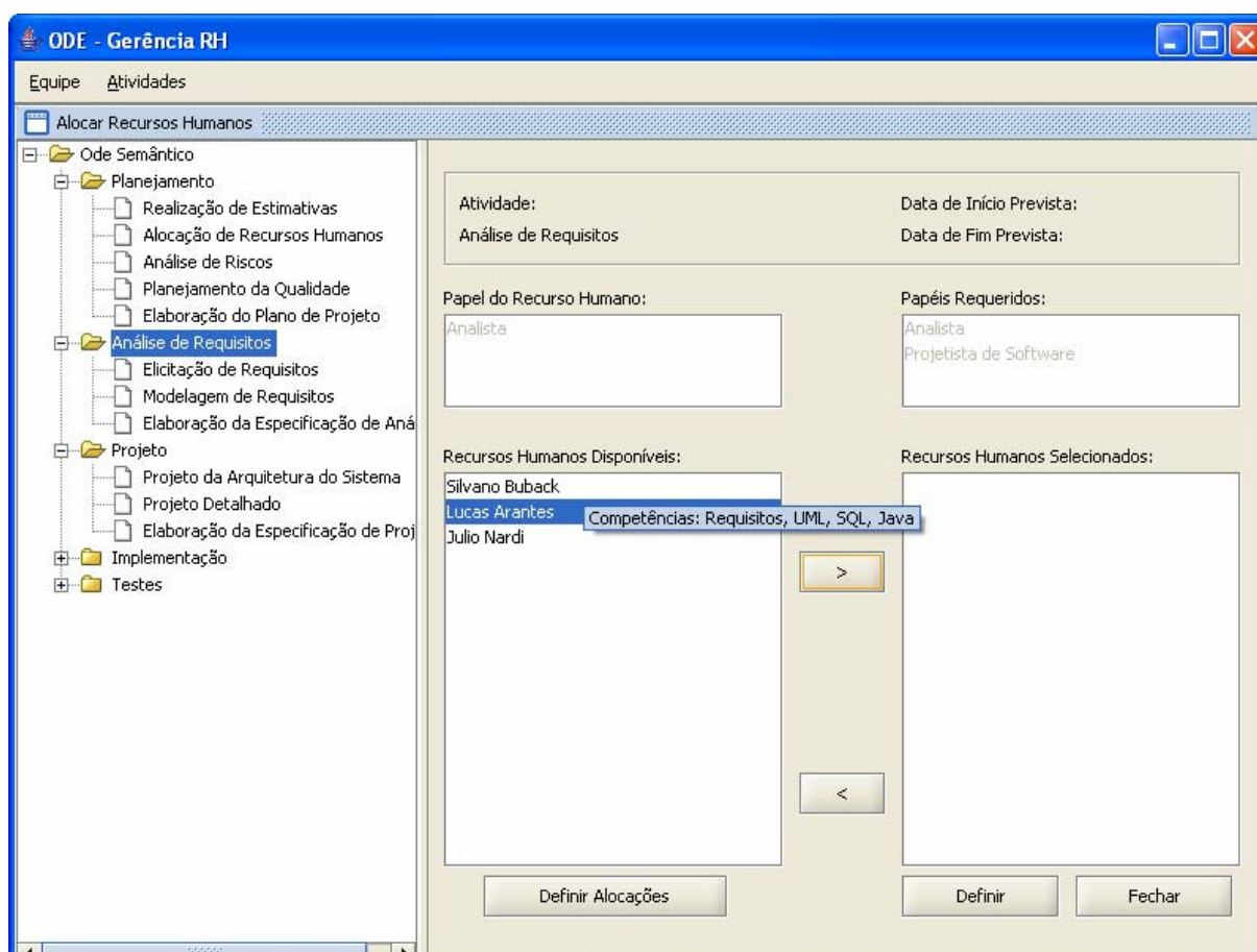
Figura 4.14 – Ferramenta GerênciaRH
