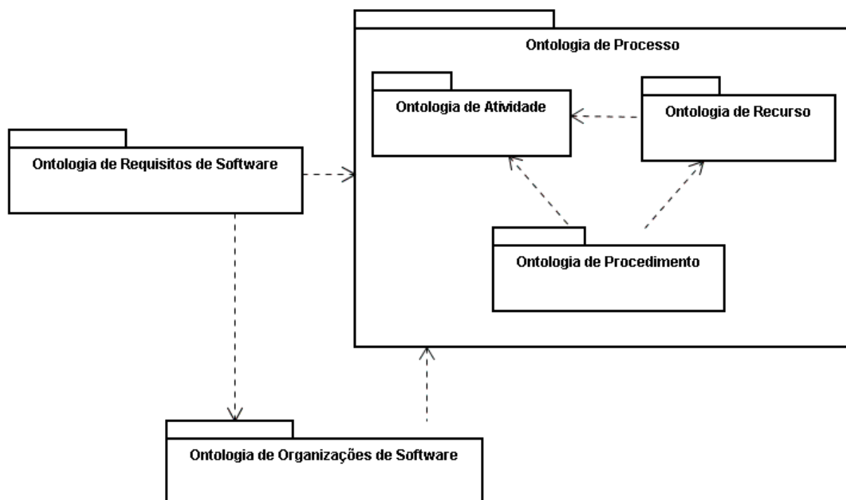
Figura 4.2 – A Ontologia de Organizações de Software e suas Relações com as demais ontologias da Base Ontológica de ODE
