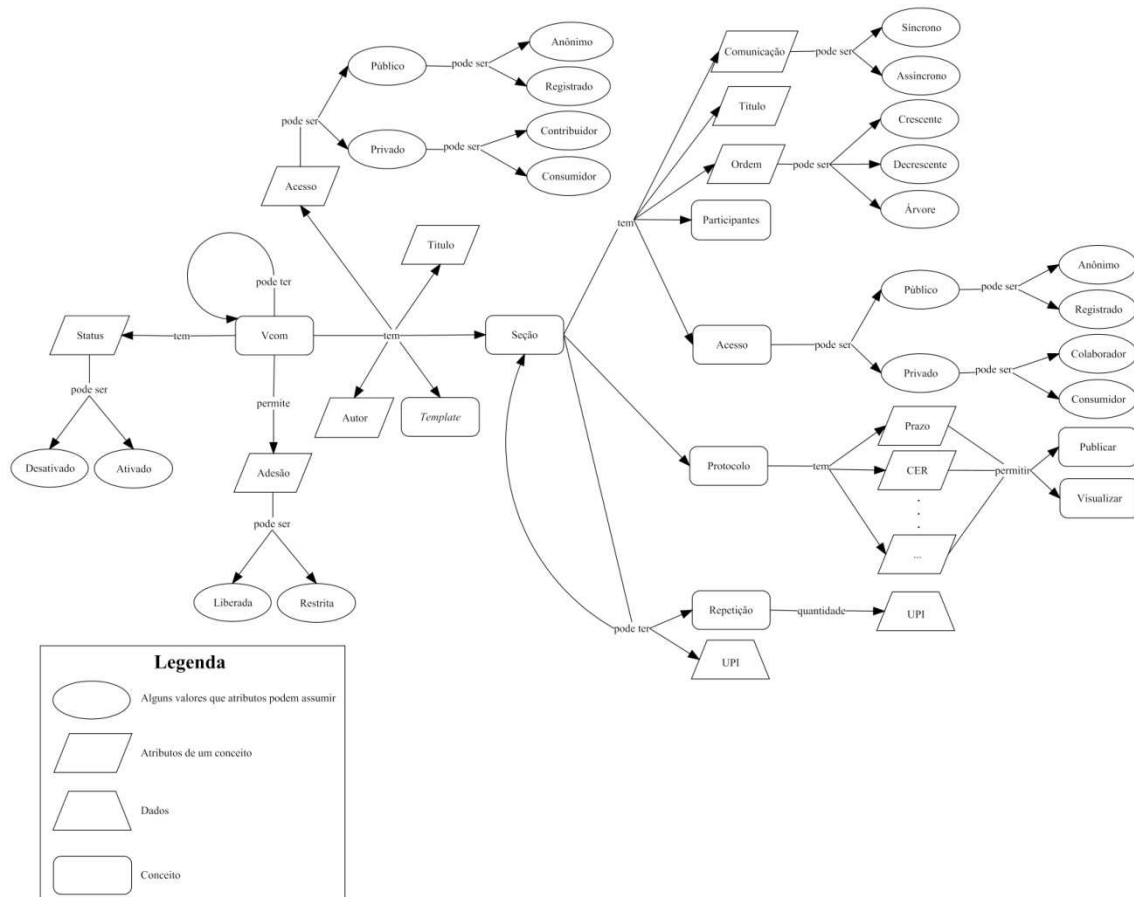
Figura 4.5 - Uma representação da estrutura de um Vcom
