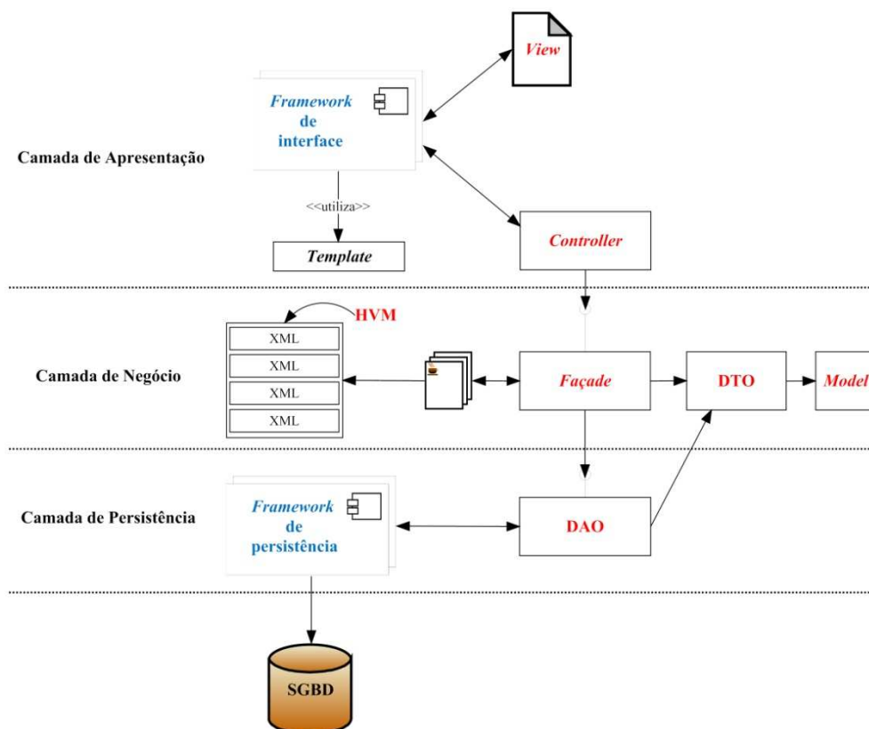
Figura 5.8 - Arquitetura Geral Interna do FrameColab
