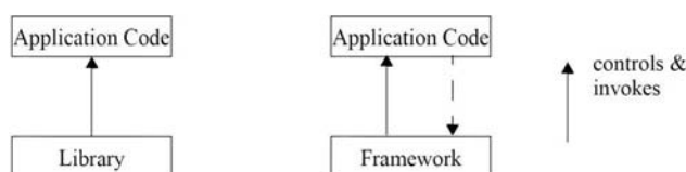
Figura 2.4 - Ilustração da inversão de controle em frameworks (Mattsson, 2000)
