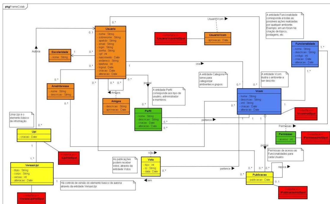
Figura 5.10 - Diagrama de classes de domínio do FrameColab. Em vermelho os hot-spots , em azul as classes pertencentes ao pacote vcom, em amarelo as classes pertencentes ao pacote producao, em
