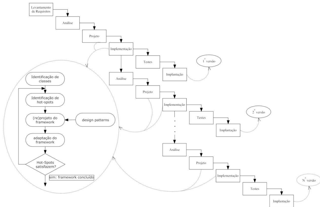
Figura 5.4 - Visão geral da metodologia de desenvolvimento
