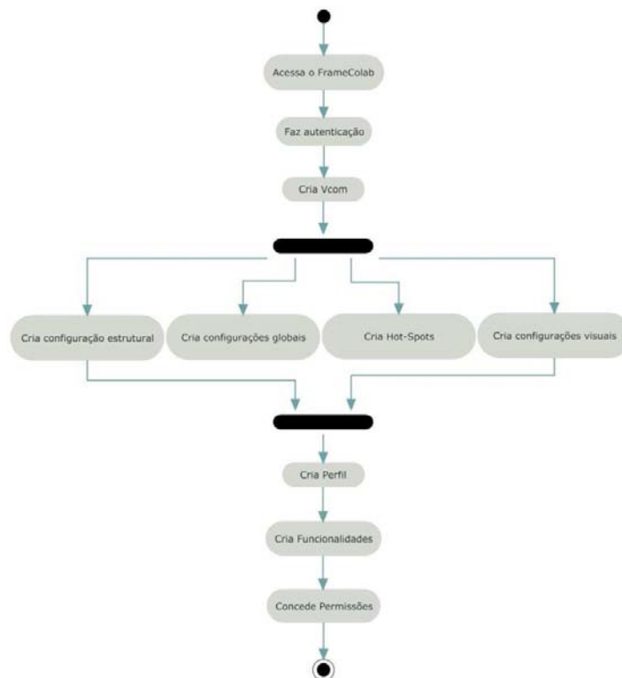
Figura 5.6 - Criação de Vcom
