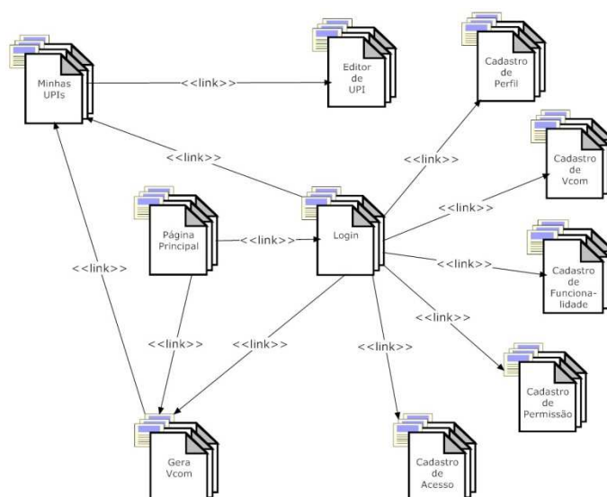
Figura 6.7 - Diagrama de navegação do protótipo do FrameColab
