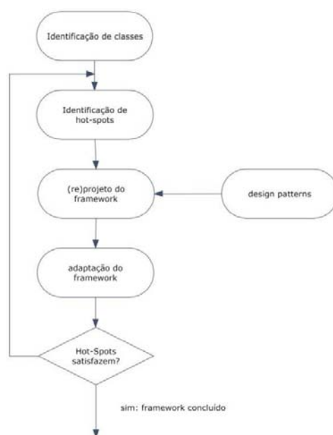
Figura 2.9 - Projeto Dirigido por Hot-Spot . Adaptado de (Pree, 1994)
