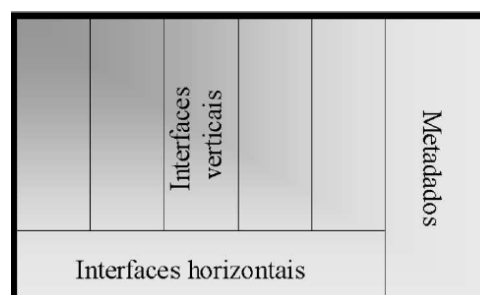
Figura 2.2 - Ilustração do HVM. Adaptado de (Mowbray & Malveau, 1997)
