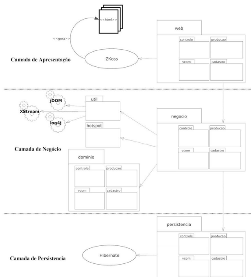
Figura 6.1 - Diagrama de artefatos do protótipo
