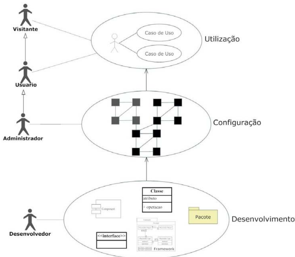
Figura 5.5 - Visão conceitual (atores x papéis). Adaptado de (Natali & Menezes, 2010)
