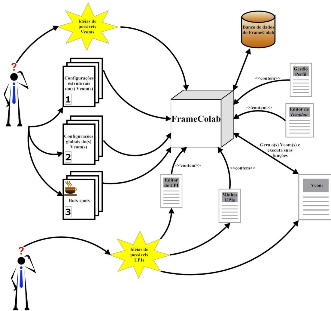
Figura 5.1- Visão geral de funcionamento do FrameColab
