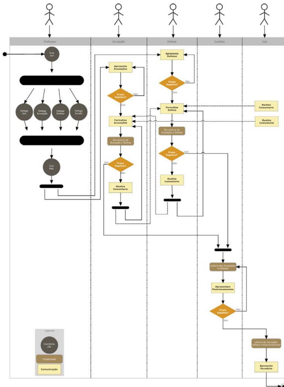
Figura 6.22 - Diagrama de atividades de um Júri Simulado exemplo
