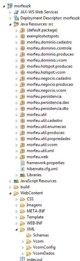
Figura 6.14 - Projeto Web Java no Eclipse do protótipo do FrameColab
