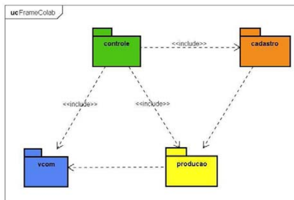
Figura 5.9 - Pacotes no FrameColab
