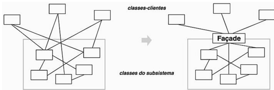
Figura 2.1 - Ilustração de uso de façade . Adaptado de (Gamma, Helm, Johnson, & Vlissides, 1994)
