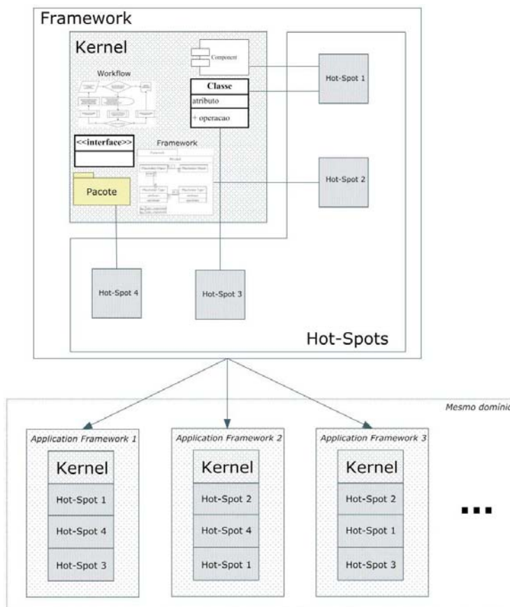
Figura 2.3 - Visão geral das partes básicas de um framework
