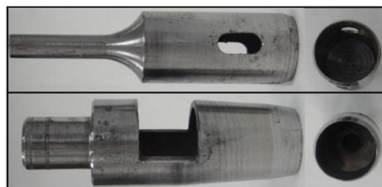
Figura 23: Comparação entre as ferramentas de corte, LFS – USP e TRICORRMAT – UFES. Fonte: Pelo próprio autor, 2012.
